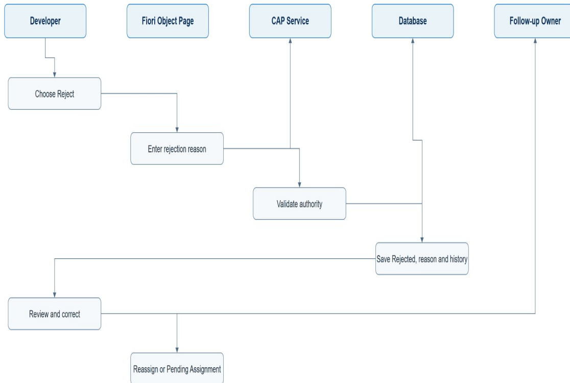
Figure 15. Rejected Follow-up Flow. IDTS Diagram Pack; bản có thể chỉnh sửa được quản lý dưới dạng file draw.io cùng artifact của dự án.
