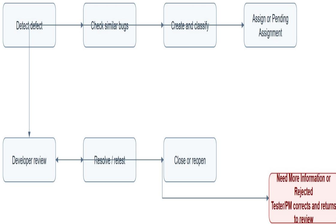
Figure 14. Main Defect Tracking Flow. IDTS Diagram Pack; bản có thể chỉnh sửa được quản lý dưới dạng file draw.io cùng artifact của dự án.
