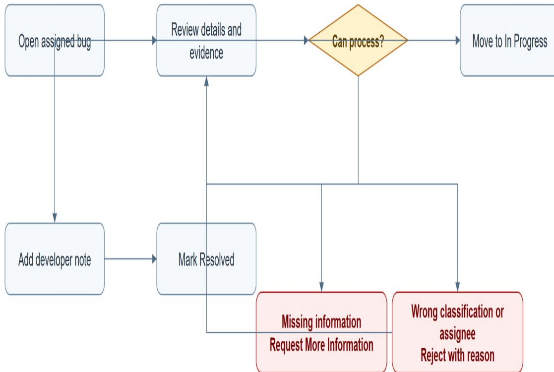
Figure 18. Developer review. IDTS Diagram Pack; bản có thể chỉnh sửa được quản lý dưới dạng file draw.io cùng artifact của dự án.
