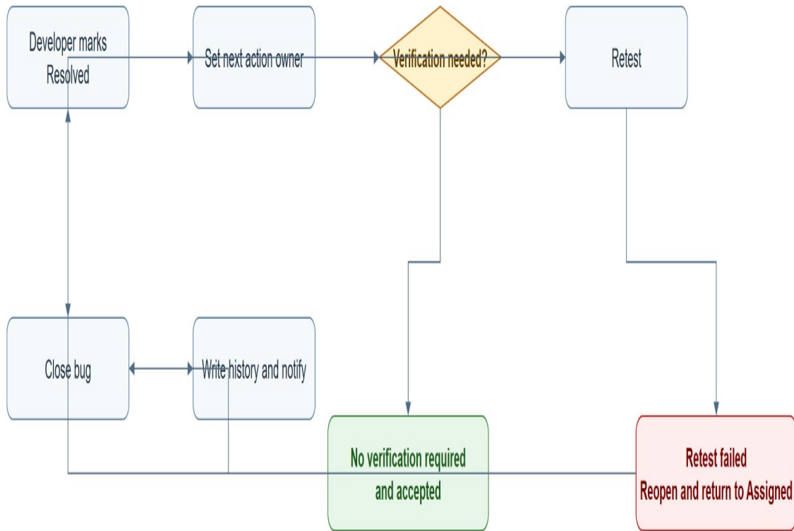
Figure 20. Resolve, retest, close và reopen. IDTS Diagram Pack; bản có thể chỉnh sửa được quản lý dưới dạng file draw.io cùng artifact của dự án.
