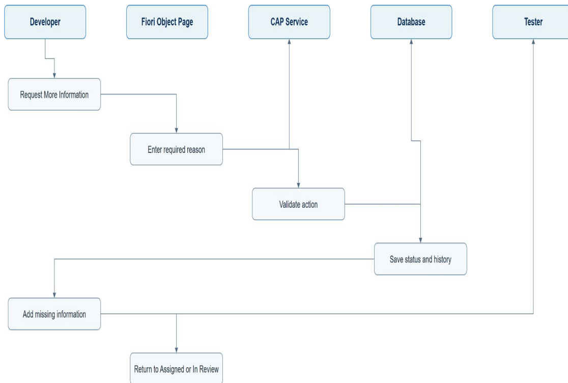
Figure 19. Request More Information Flow. IDTS Diagram Pack; bản có thể chỉnh sửa được quản lý dưới dạng file draw.io cùng artifact của dự án.
