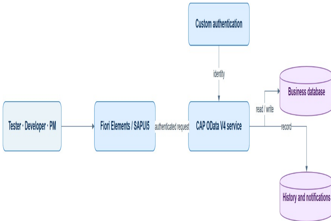
Figure 13. Bối cảnh hệ thống SRS. IDTS Diagram Pack; bản có thể chỉnh sửa được quản lý dưới dạng file draw.io cùng artifact của dự án.
