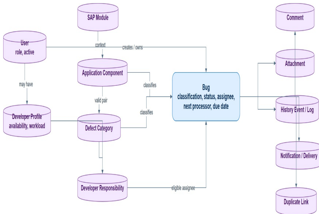
Figure 09. Mô hình dữ liệu IDTS khái niệm. IDTS Diagram Pack; bản có thể chỉnh sửa được quản lý dưới dạng file draw.io cùng artifact của dự án.
