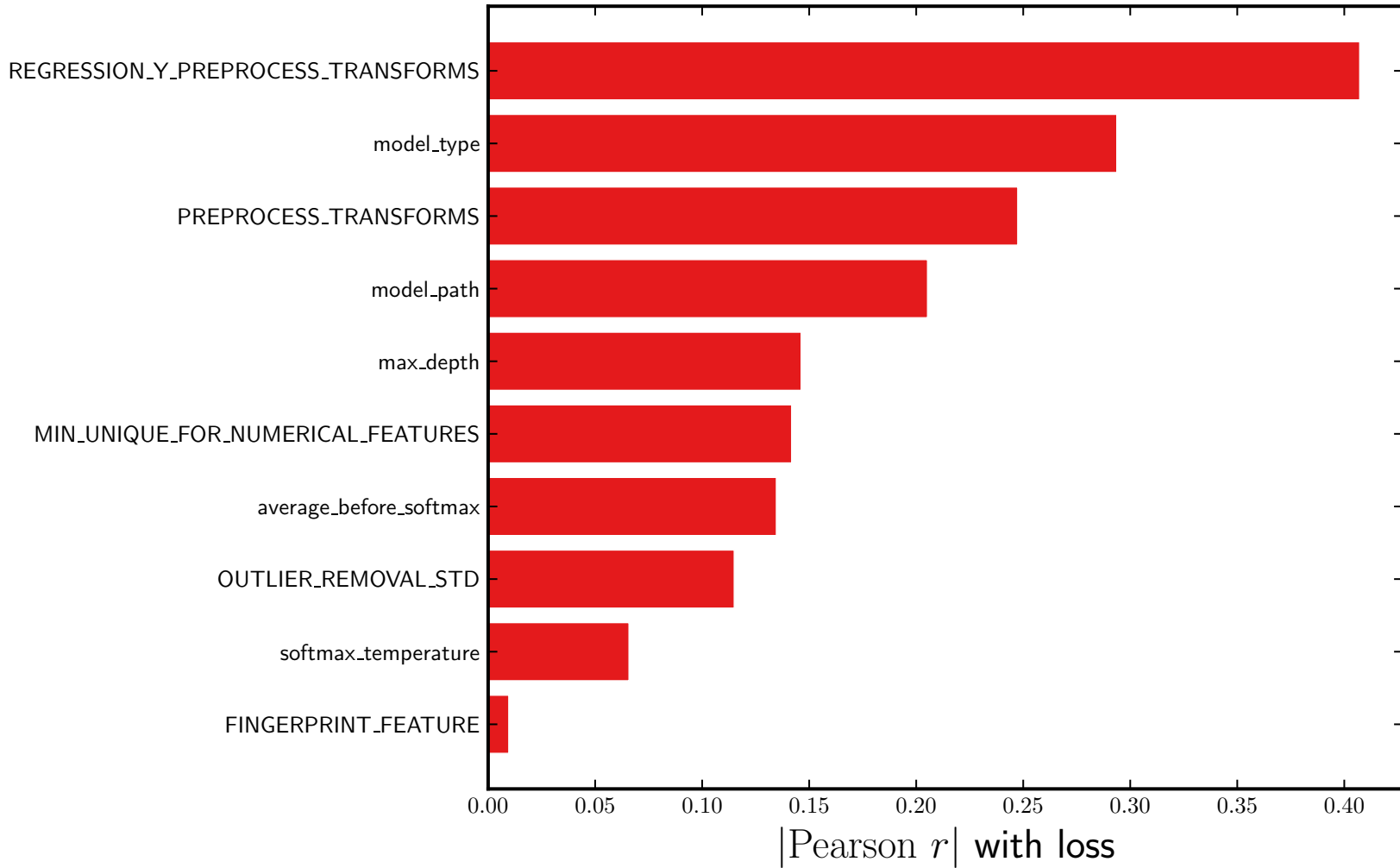
Hyperparameter
