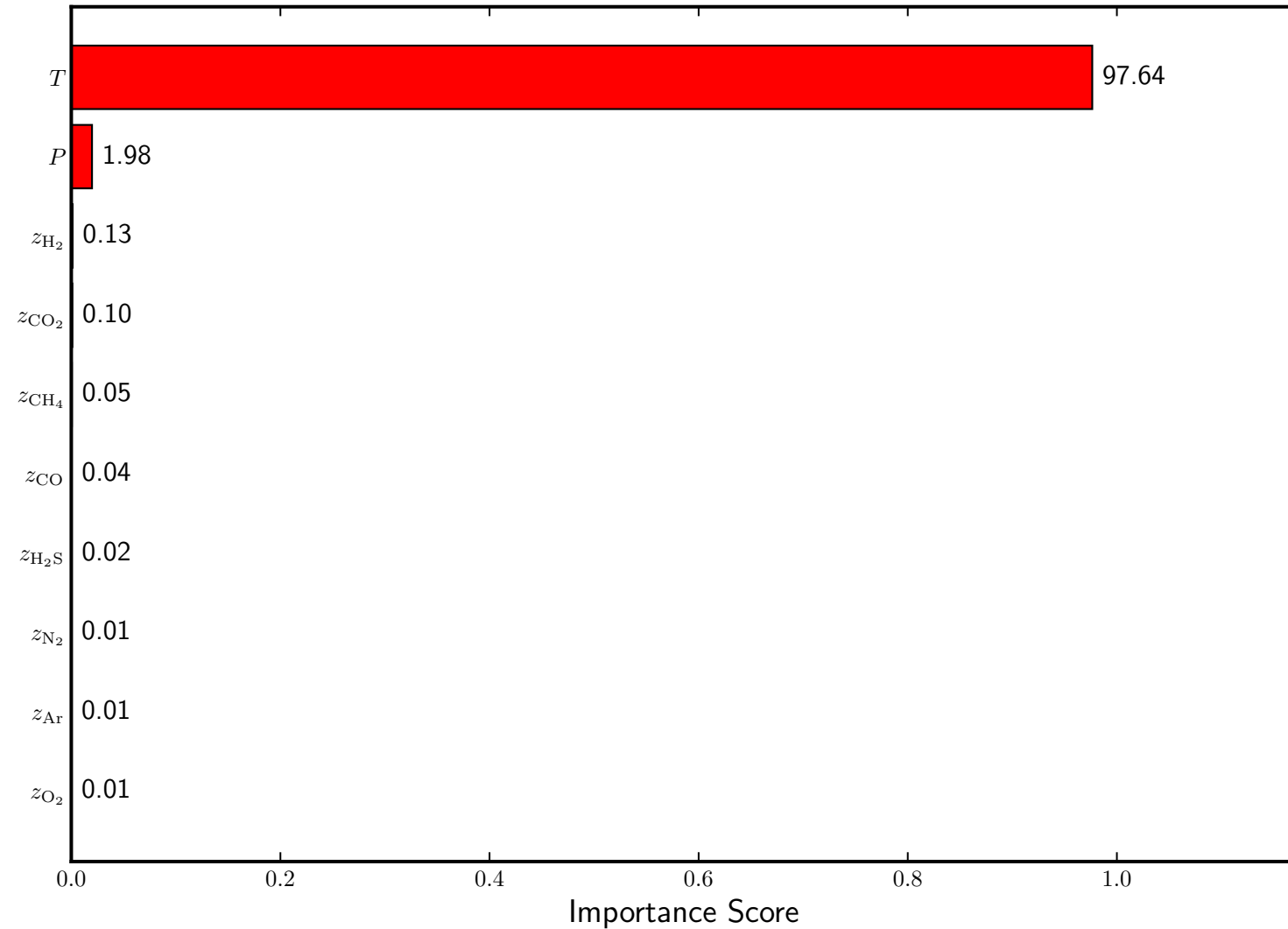
Feature Importance (Linear Scale)
