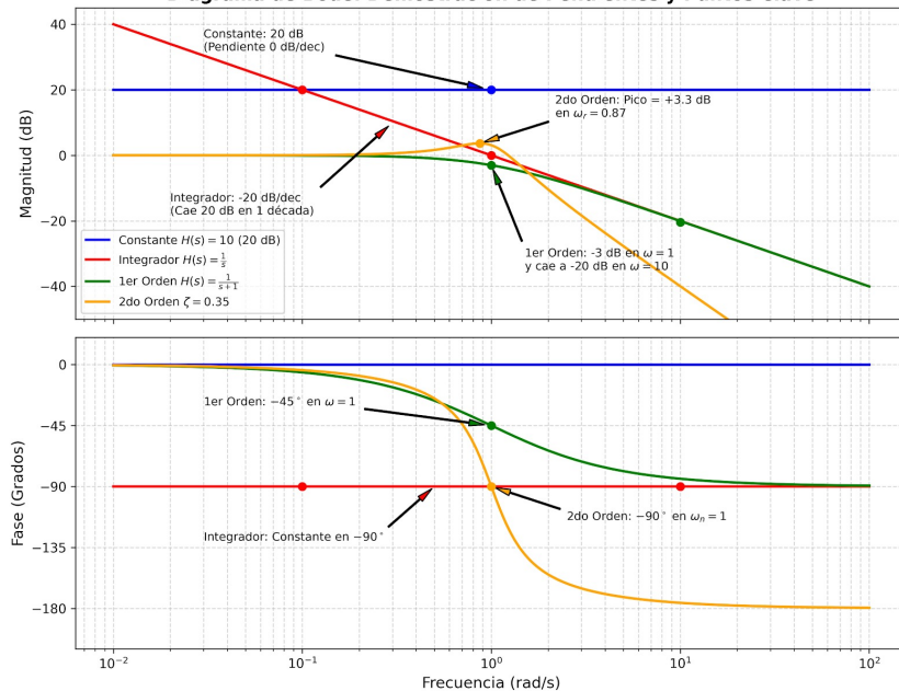
Diagrama de Bode: Demostración de Pendientes y Puntos Clave
