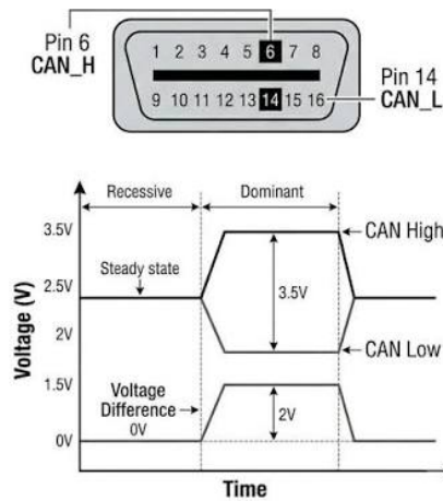
Fig. 2: Niveles de voltaje diferencial: estado dominante vs recesivo
