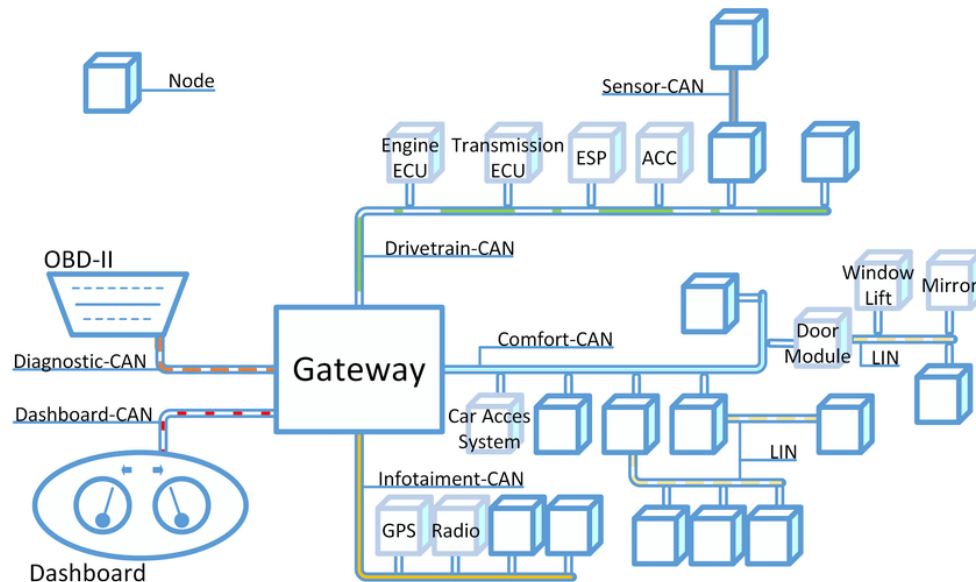
Fig. 6: Ejemplo de red vehicular con múltiples buses CAN interconectados mediante un gateway
