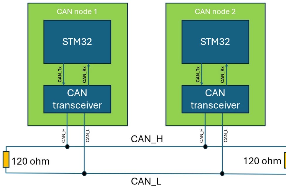
Fig. 7: Esquemático de conexión STM32 + transceptor CAN + bus terminado
