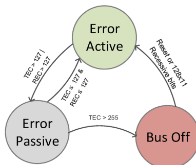
Fig. 5: Máquina de estados de confinamiento de fallas (fault confinement)
