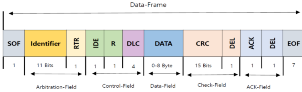
Fig. 4: Estructura completa de la trama de datos CAN estándar (CAN 2.0A)
