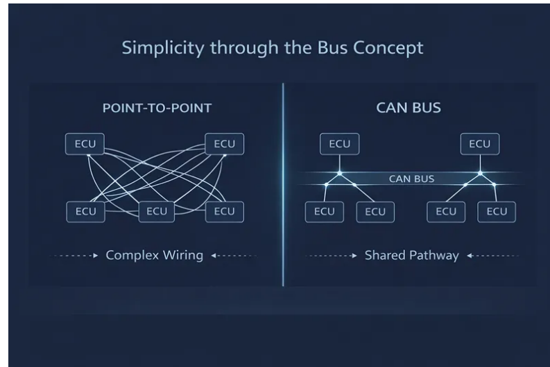
Fig. 1: Comparación entre cableado punto a punto tradicional y topología de bus CAN
