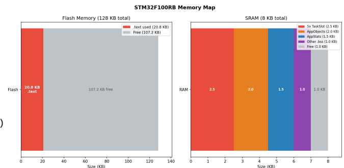
Fig. 14. Memory Map
