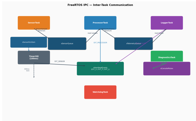
Fig. 3. Ipc Diagram
