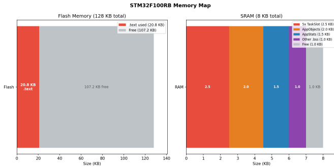
Fig. 13. Memory Map
