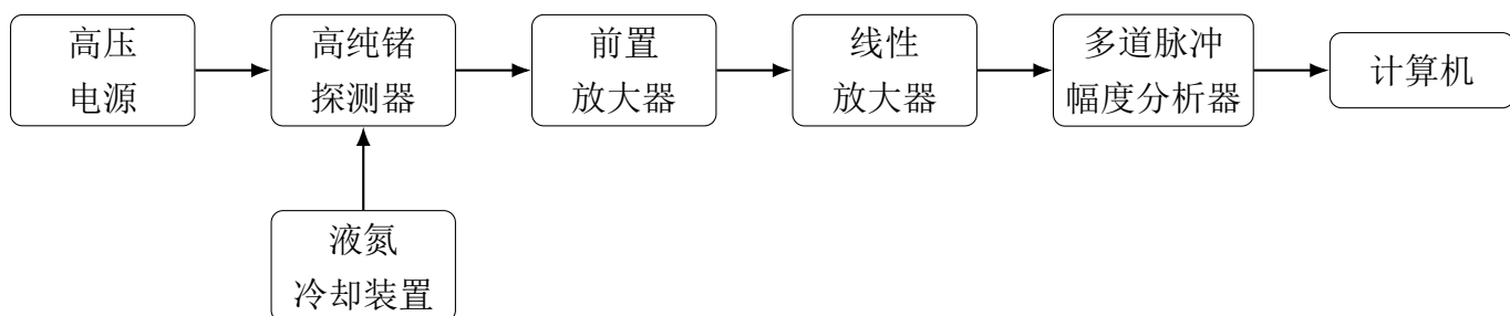
图 2: 高纯锗 \gamma 谱仪方框图
