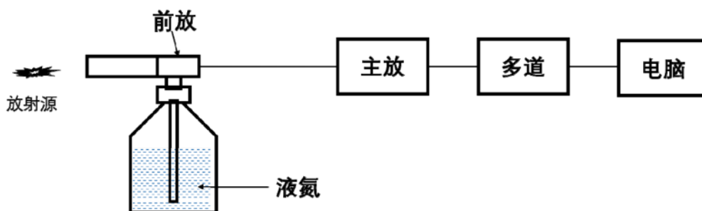
图 2: 高纯锗 \gamma 谱仪方框图
