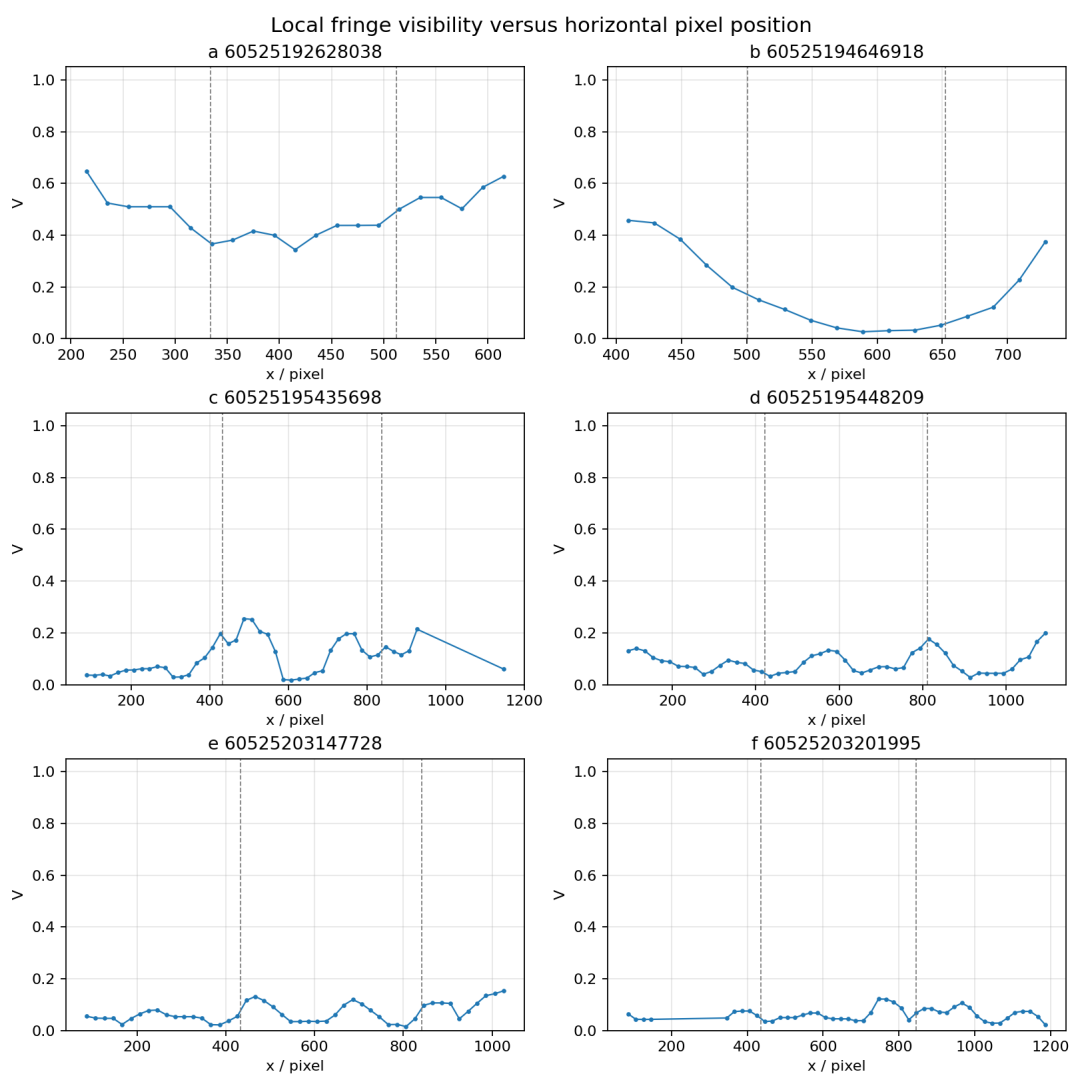
图 6: 由实验图像提取的局部条纹可见度 V(x)
