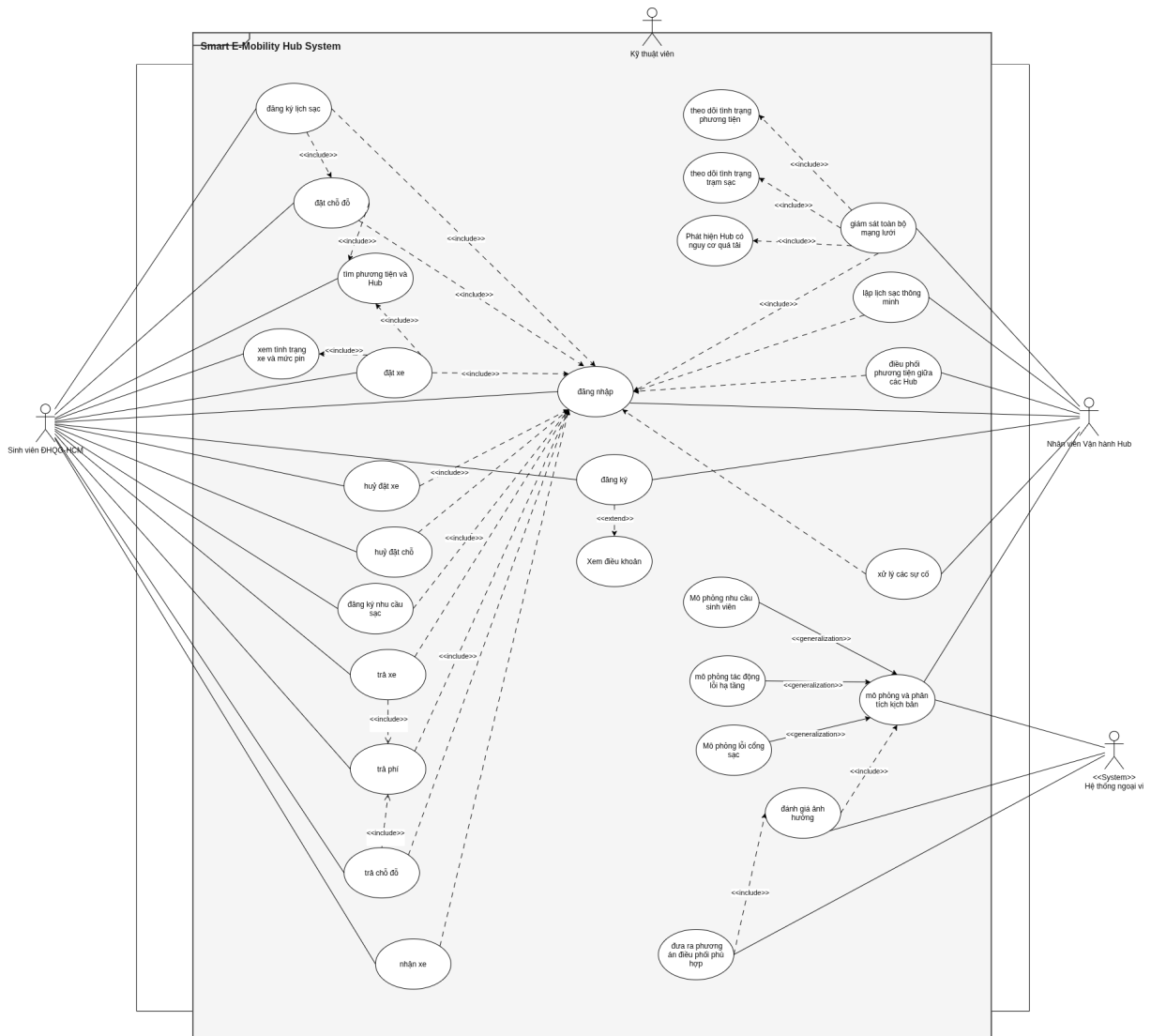
Hình 2.1: Sơ đồ Use-Case Tổng thể của Hệ thống Smart E-Mobility Hub
