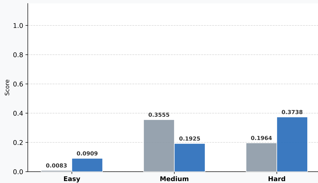
Context Precision
