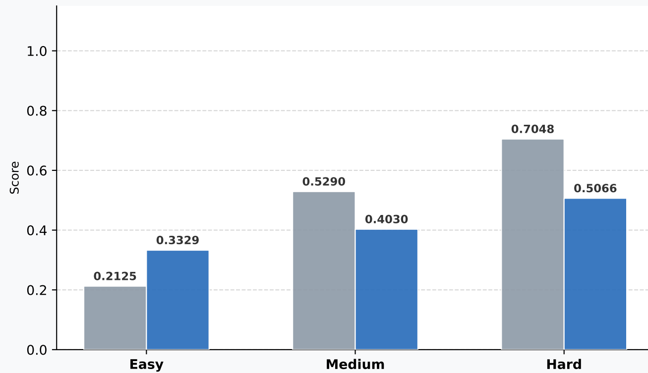
Context Precision
