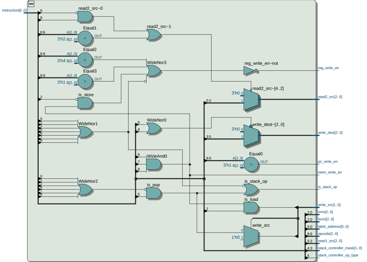
decoder:decoder_inst
