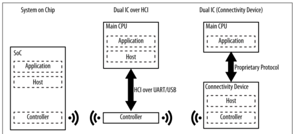
Hình 2.2: Kiểu cấu hình phần cứng chính của 1 thiết bị Bluetooth
