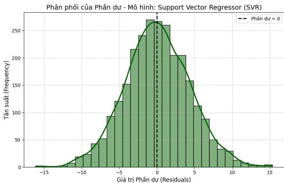
Hình 4.8: Biểu đồ phân phối của phần dư
