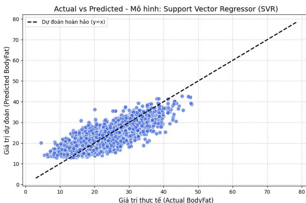
Hình 4.6: Biểu đồ thể hiện các giá trị tương quan giữa Thực tế và Dự đoán
