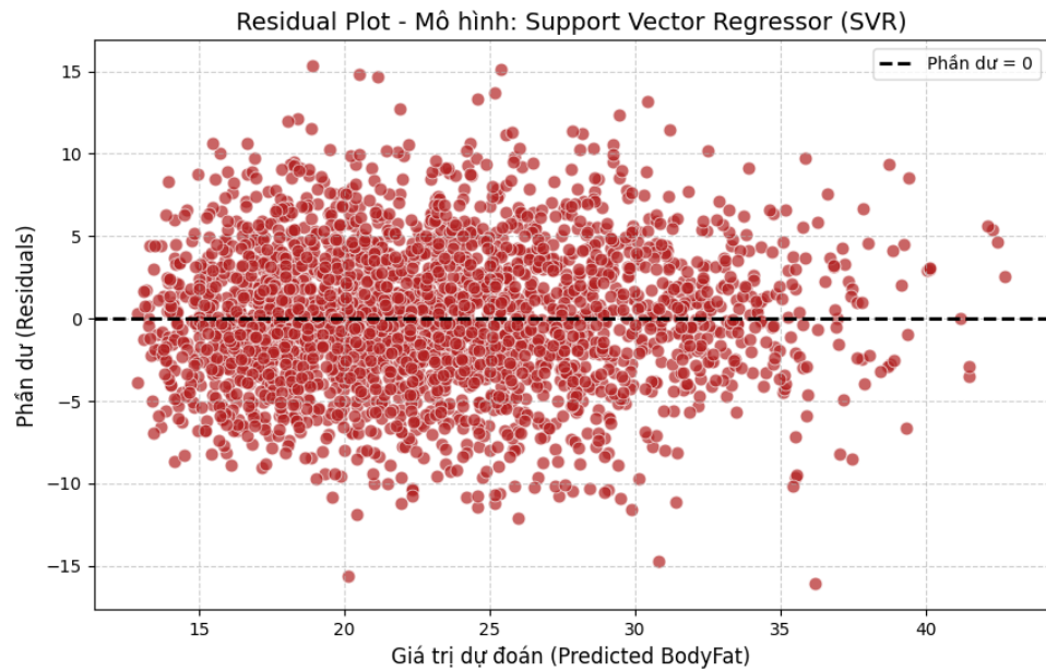
Hình 4.7: Biểu đồ phần dư
