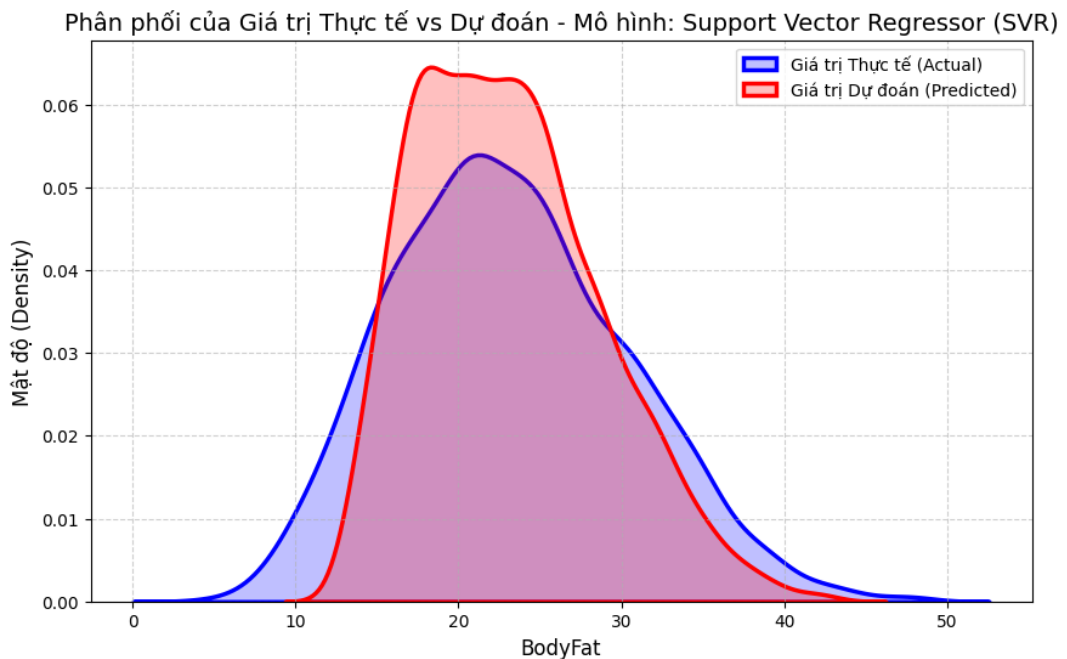
Hình 4.11: Biểu đồ phân phối của giá trị thực tế và dự đoán
