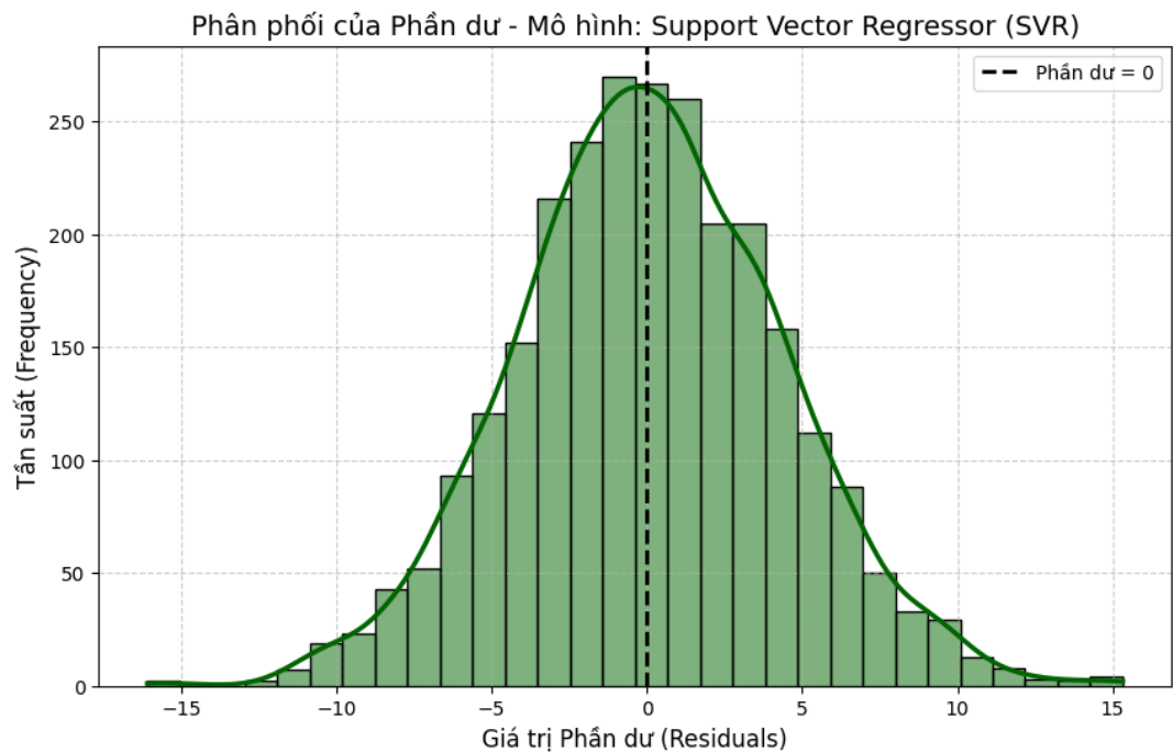
Hình 4.10: Biểu đồ phân phối của phần dư
