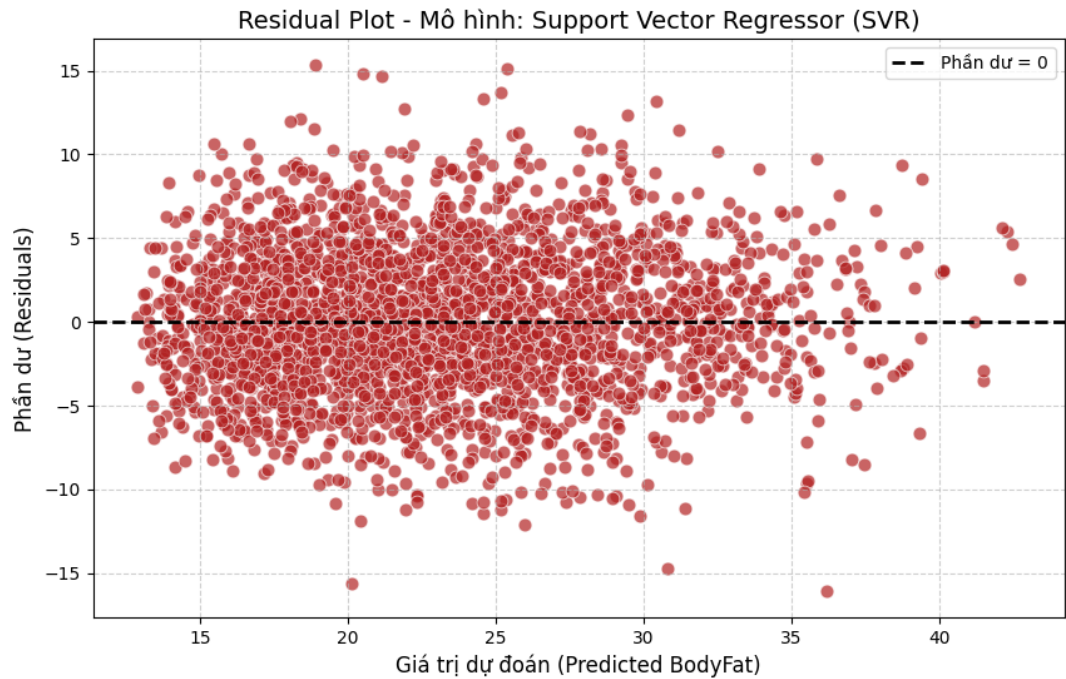
Hình 4.9: Biểu đồ phần dư
