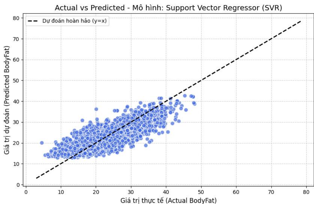
Hình 4.8: Biểu đồ thể hiện các giá trị tương quan giữa Thực tế và Dự đoán
