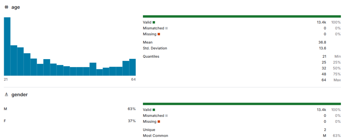
Hình 3.5: Thông tin độ tuổi và giới tính có trong bộ dữ liệu được huấn luyện để dự đoán tỷ lệ phần trăm mỡ trong cơ thể
