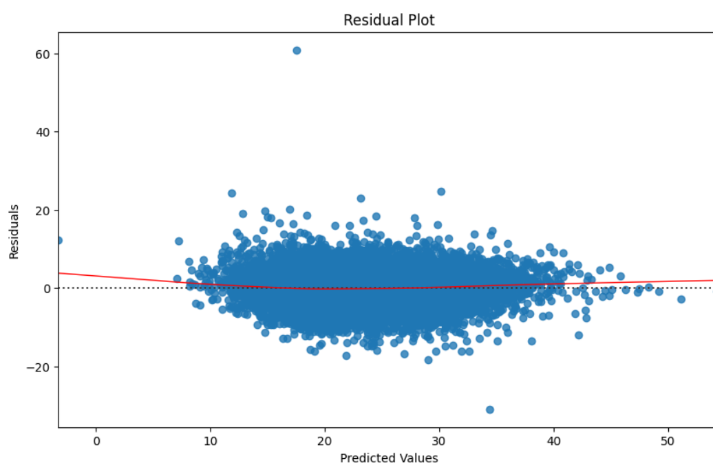
Hình 4.8: Biểu đồ phần dư
