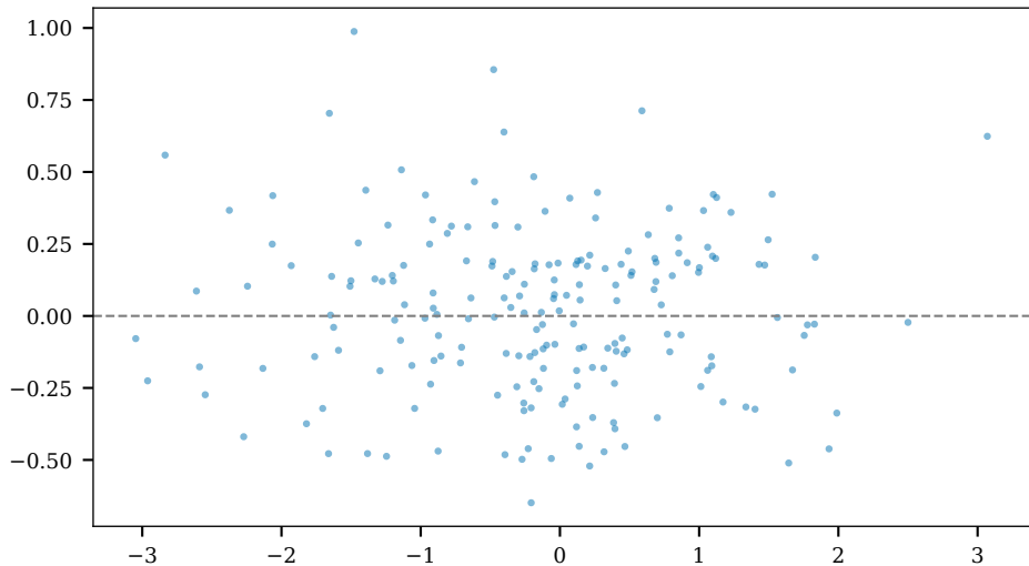
Parameter Recovery
