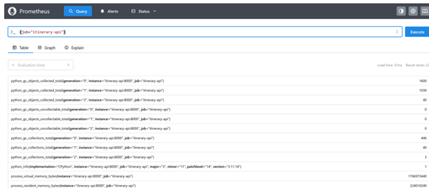
Prometheus Query exemple sur job="itinerary-api"
