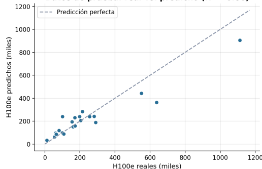
Datos de prueba: real vs. predicho ( R^2 = 0.86 )
