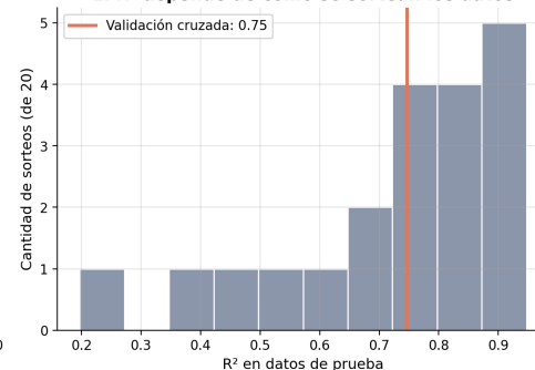
El R^2 depende de cómo se sortean los datos
