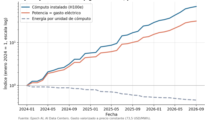
Paradoja de Jevons: cada chip gasta menos, pero se instalan muchísimos más
