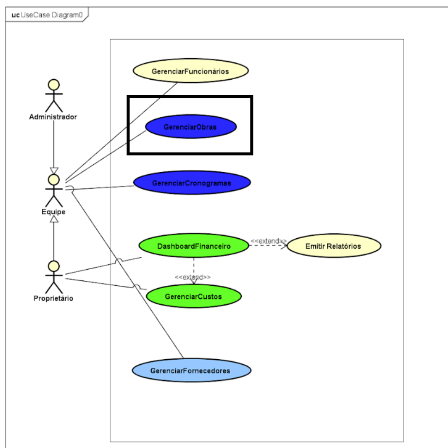
Figura 1 - Implementação do caso de uso no diagrama.
