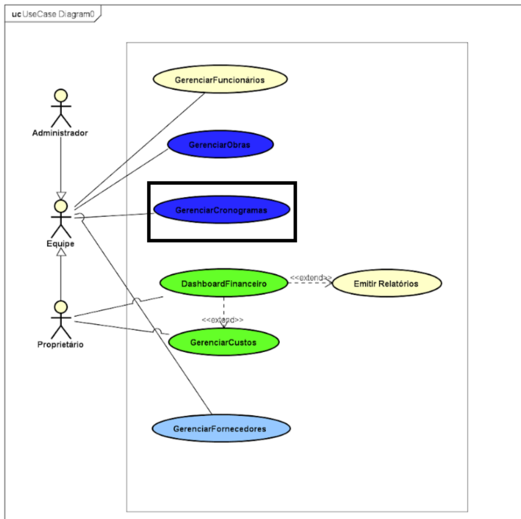
Figura 1 - Implementação do caso de uso no diagrama.
