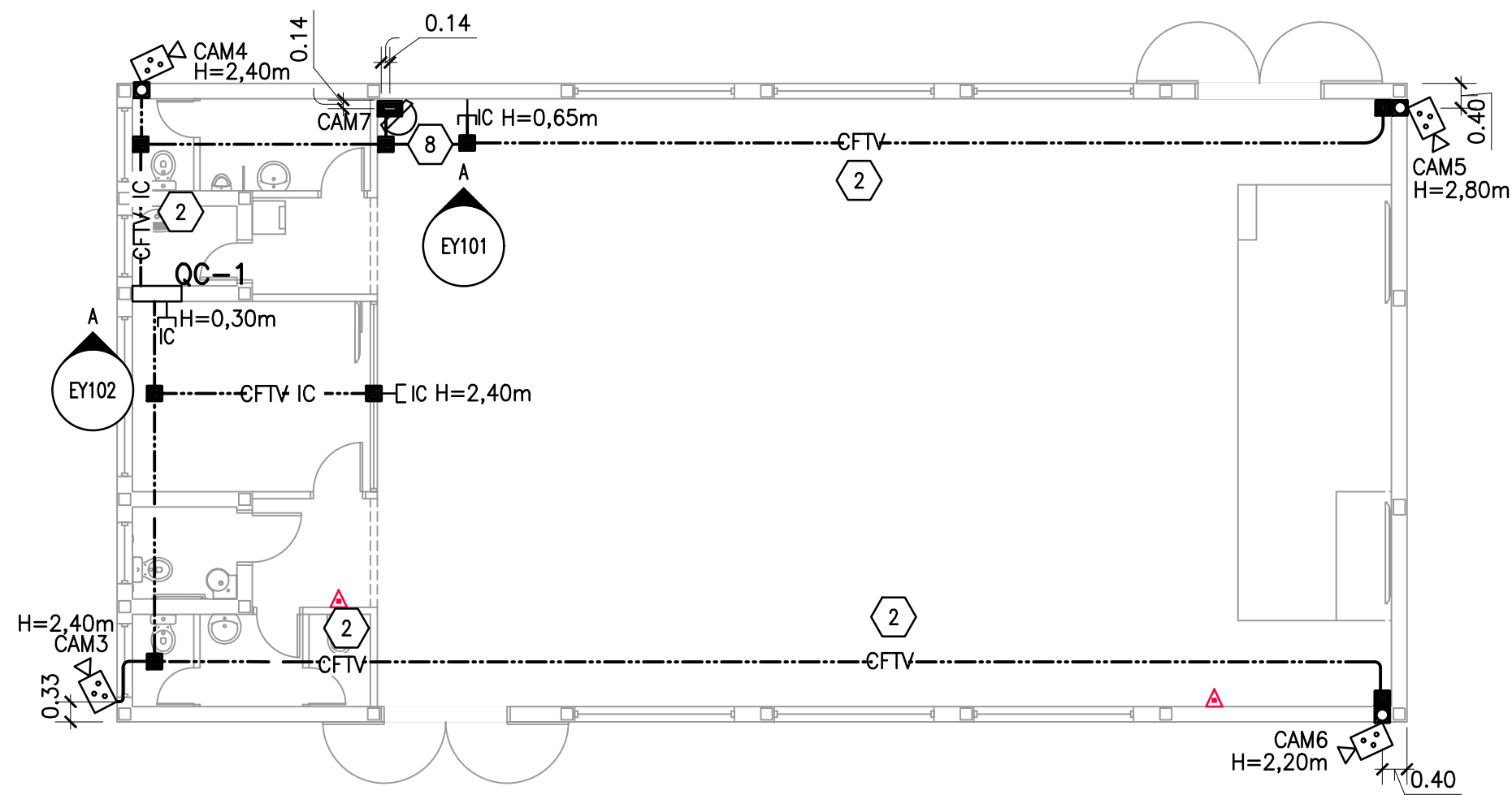
2 PLANTA BAIXA SISTEMA DE CFTV E REDE DE DADOS
