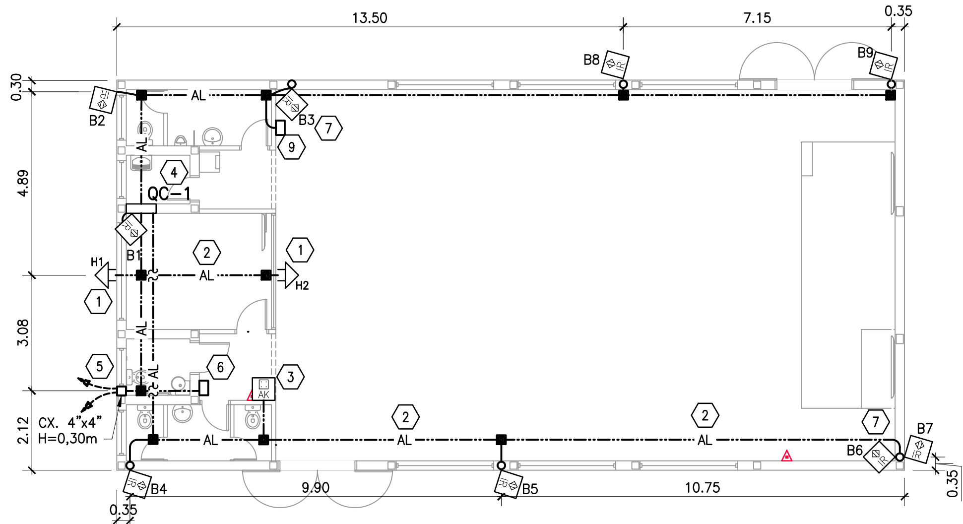
1 PLANTA BAIXA SISTEMA DE ALARME DE INTRUSÃO
