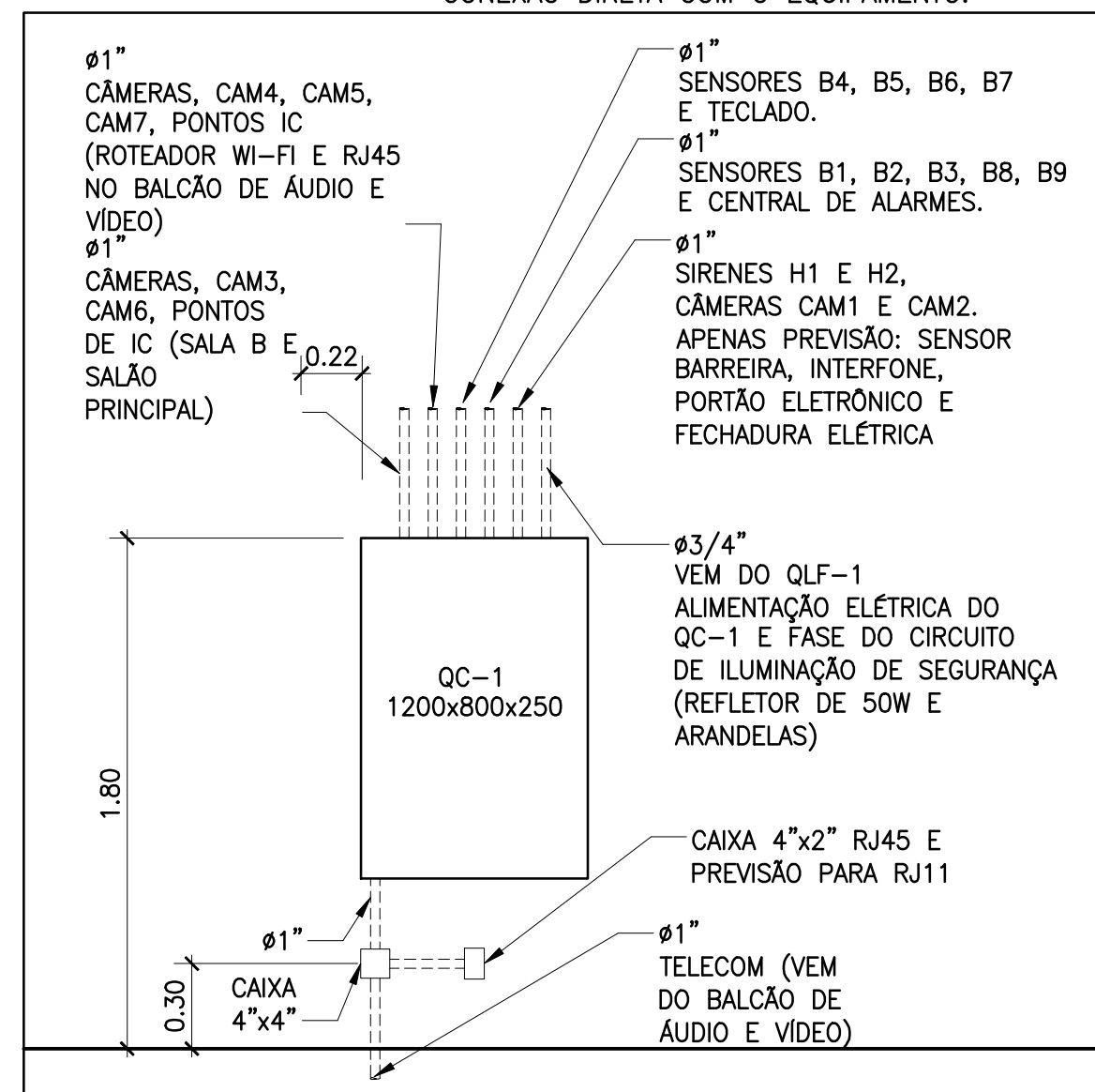
A ELEVÇÃO QUADRO QC-1
