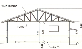
B CORTE TRANSVERSAL
