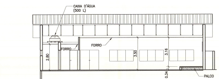
A CORTE LONGITUDINAL
