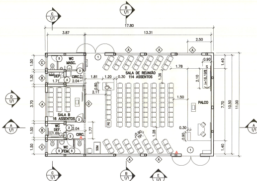
2 PLANTA BAIXA
