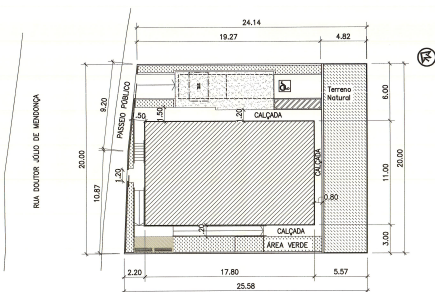
1 IMPLANTAÇÃO
