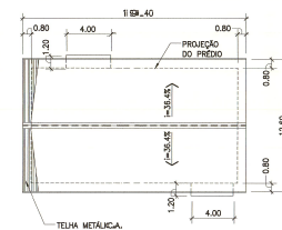
3 PLANTA DE COBERTURA
