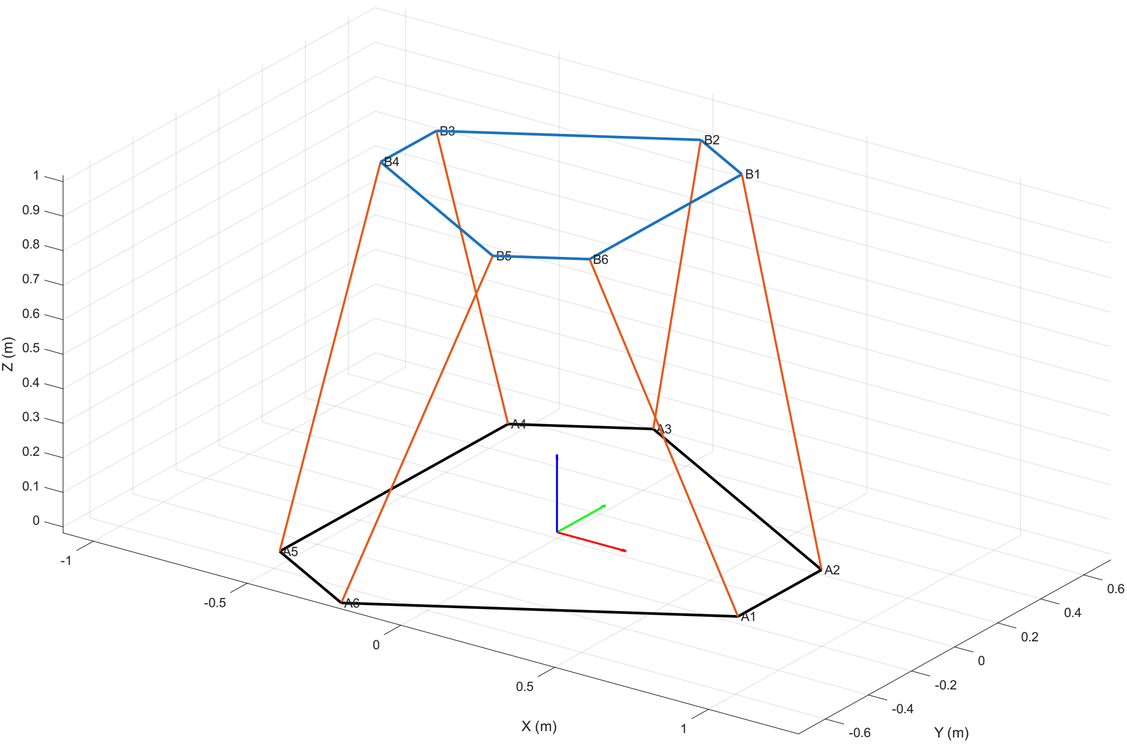
Stewart 平台几何、坐标系与六条支链
