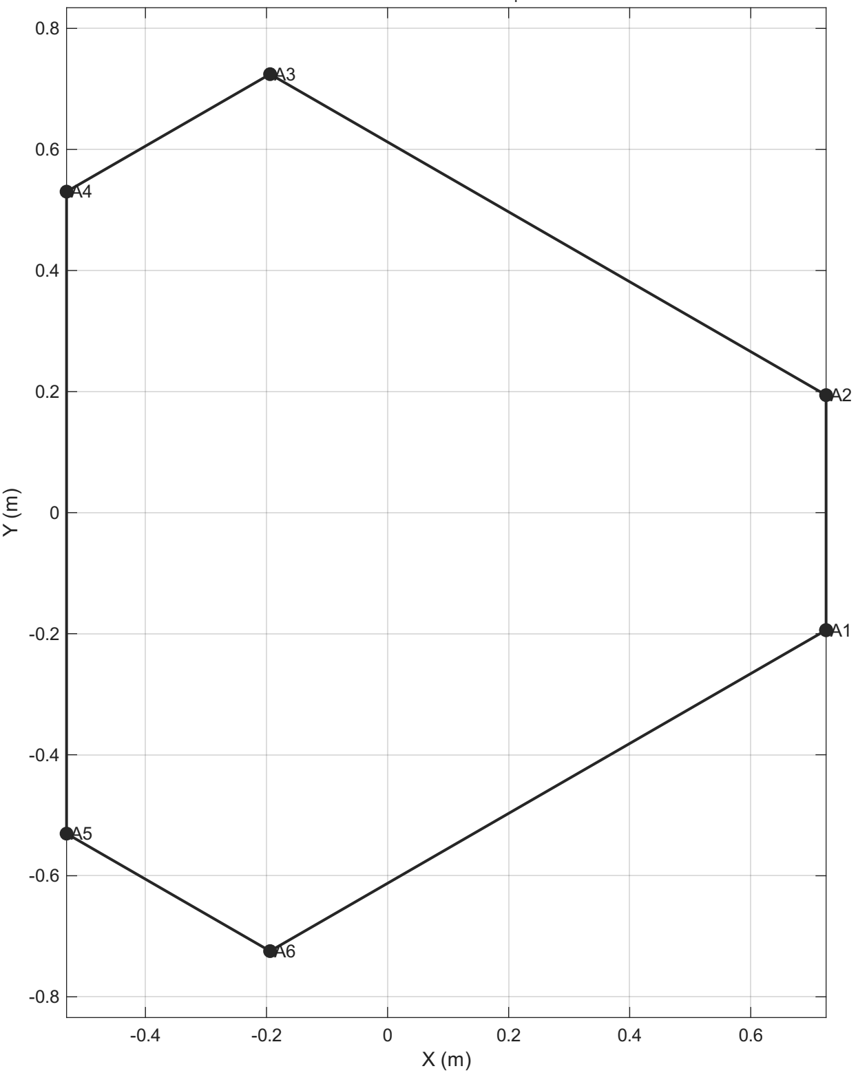
固定平台铰点 A_i
