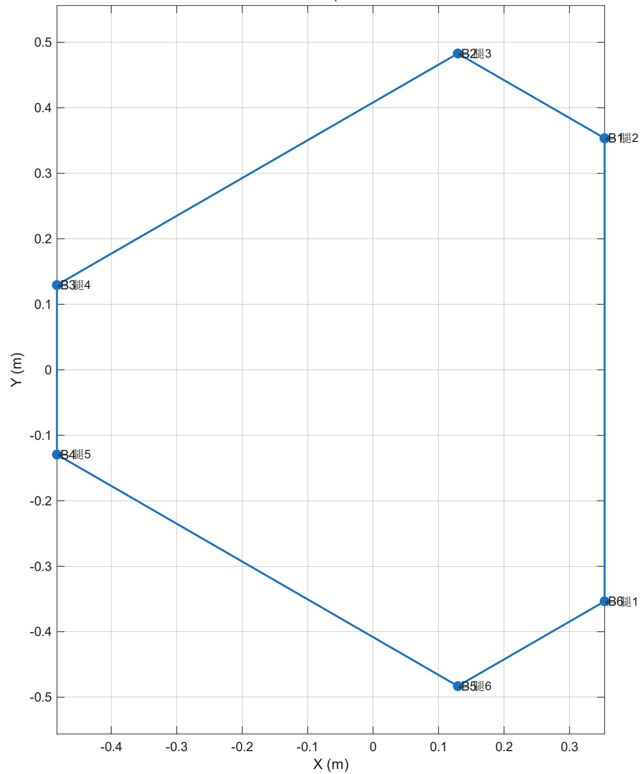
动平台铰点 B_i 与实际支链
