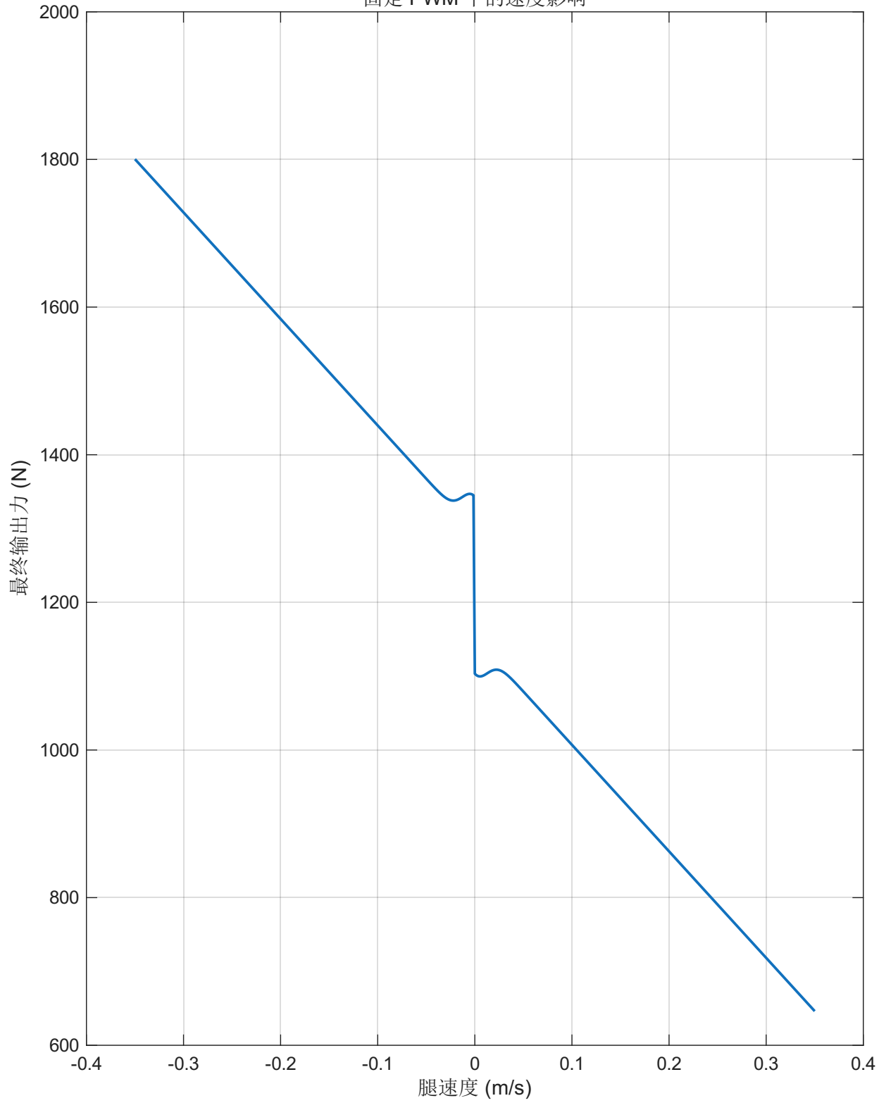
固定 PWM 下的速度影响
