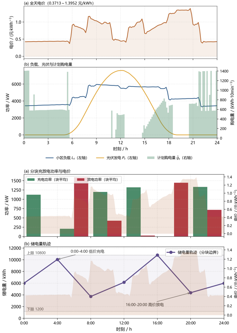
图 6 问题一：(a) 全天电价、负载、光伏与计划购电量；(b) 分块充放电功率与储电量轨迹
