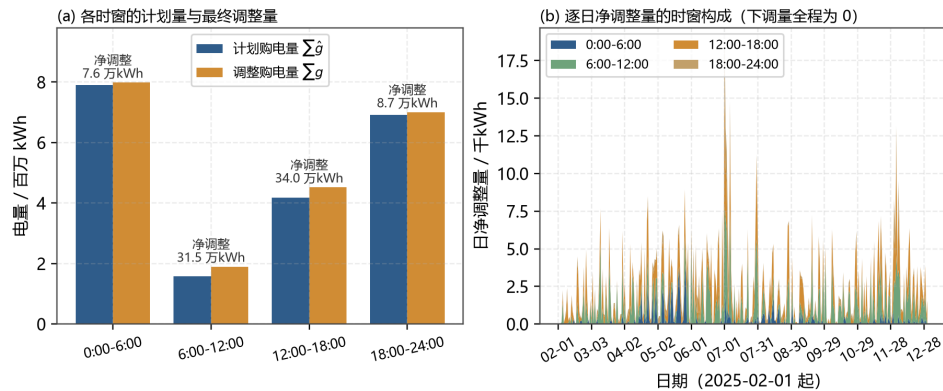
图 10 问题三：按 6 小时时窗的计划量与调整量
