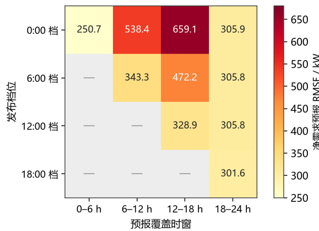
图 13 各发布档、各时窗的净需求预报 RMSE 矩阵
