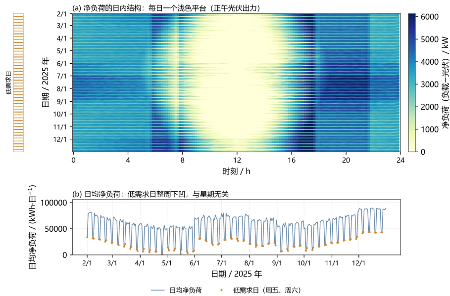
图 4 全年净负荷的日内结构与逐日水平（计费窗口 334 天；左侧细带为由暖机期推出的低需求日标记）
