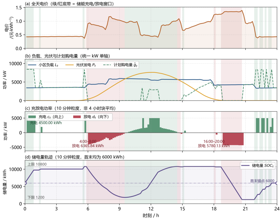
图 6 问题一的全天决策链：(a) 全天电价；(b) 负载、光伏与计划购电量；(c) 充放电功率（10 分钟粒度）；(d) 储电量轨迹。(c)(d) 的逐槽充放与储电量由问题一 LP 重解得到，其 6 个 4 小时块汇总与交付文件 result1.xlsx 逐块一致。
