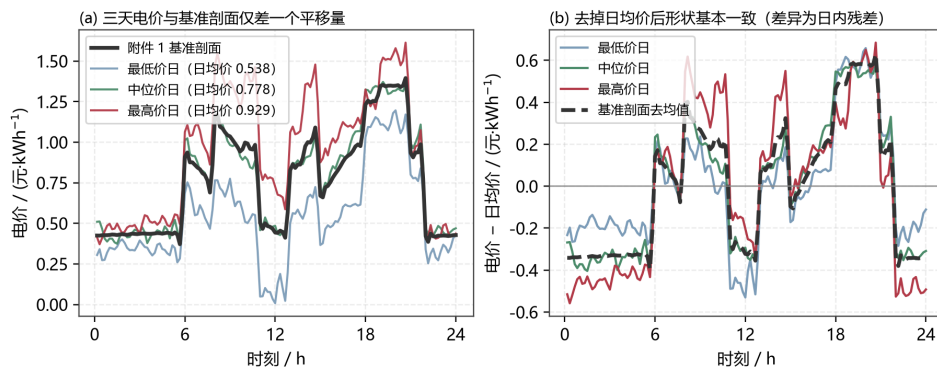
图 15 附件 4 的代表性日与基准剖面
