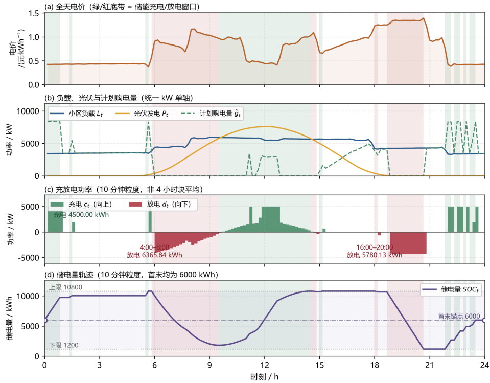
图6 问题一的全天决策链：(a) 全天电价；(b) 负载、光伏与计划购电量；(c) 充放电功率（10分钟粒度，非4小时块平均）；(d) 储电量轨迹。（c)(d)的逐槽充放与储电量由问题一LP重解得到，其6个4小时块汇总与交付文件 result1.xlsx 逐块一致。
