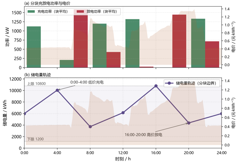
图 5 问题一：分块充放电功率与储电量轨迹
