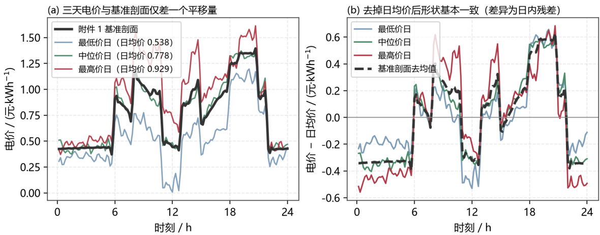
图 13 附件 4 的代表性日与基准剖面
