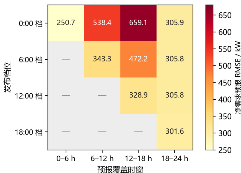
图 11 各发布档、各时窗的净需求预报 RMSE 矩阵
