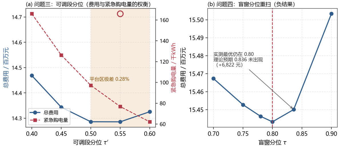
图 9 对冲分位的敏感性
