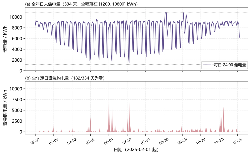
图 7 问题二：全年日末储电量与逐日紧急购电量
