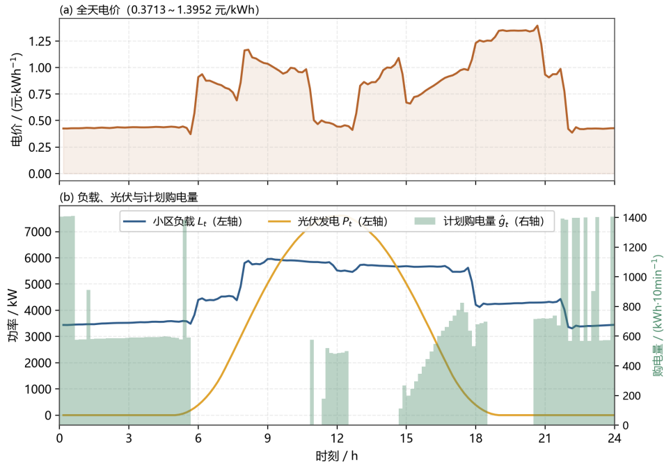
图 4 问题一：全天电价、负载、光伏与计划购电量
