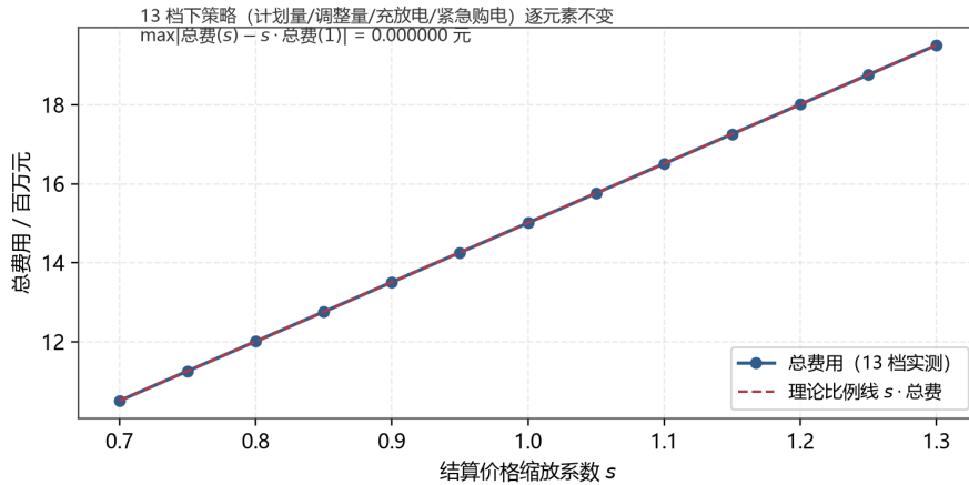
图 15 结算价格 \pm 30\% 的敏感性
