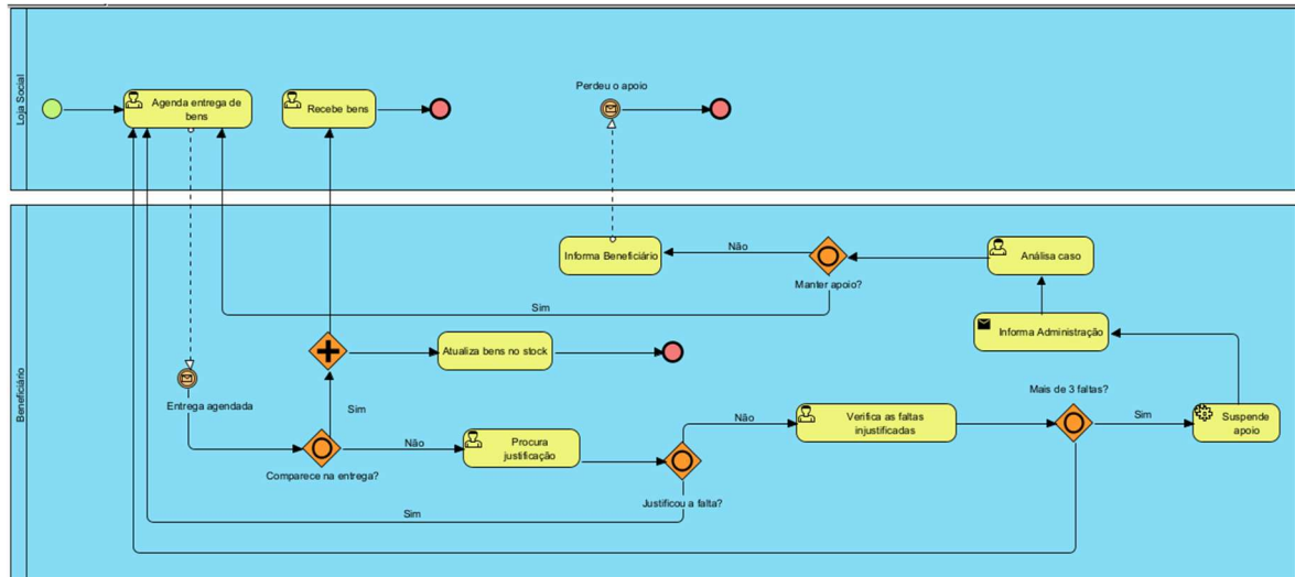
Figura 5 - Diagrama BPMN Gestão Beneficiários
