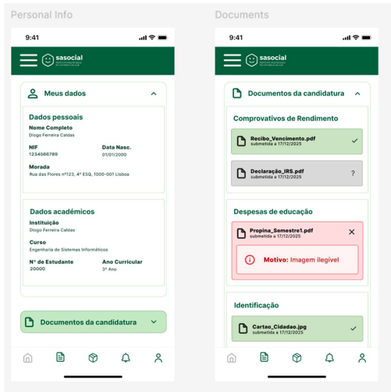
Figura 25- Mockups das páginas de dados e documentos
