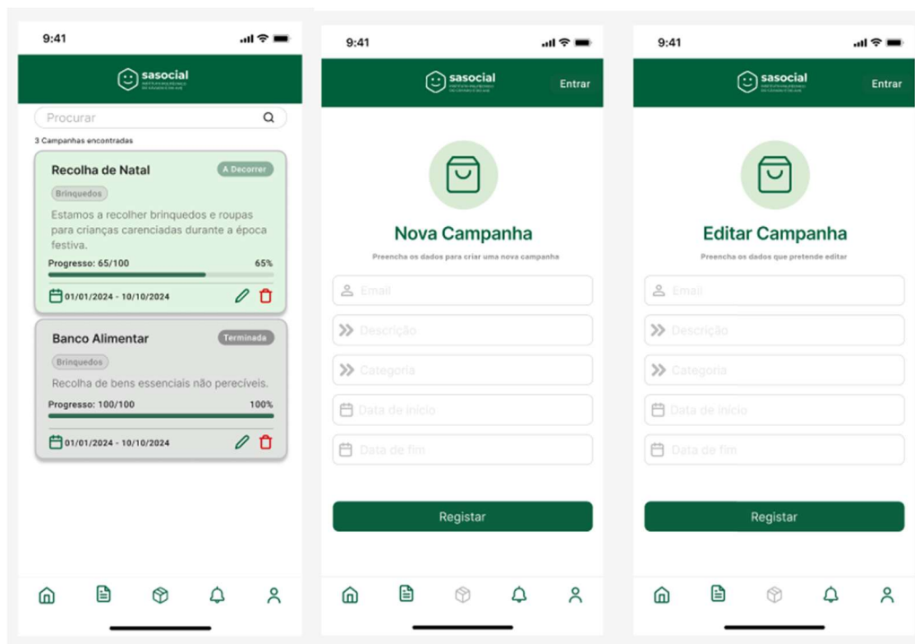
Figura 40– Mockups de gestão de campanhas
