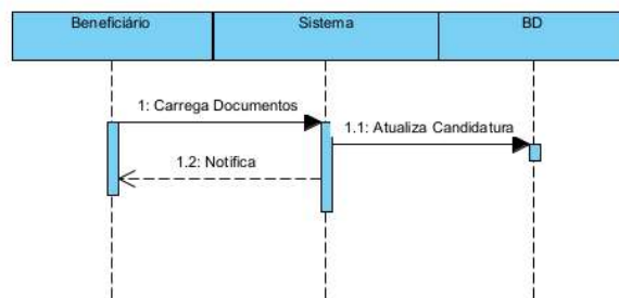
Figura 26 – Diagrama de Sequência de Documentação
