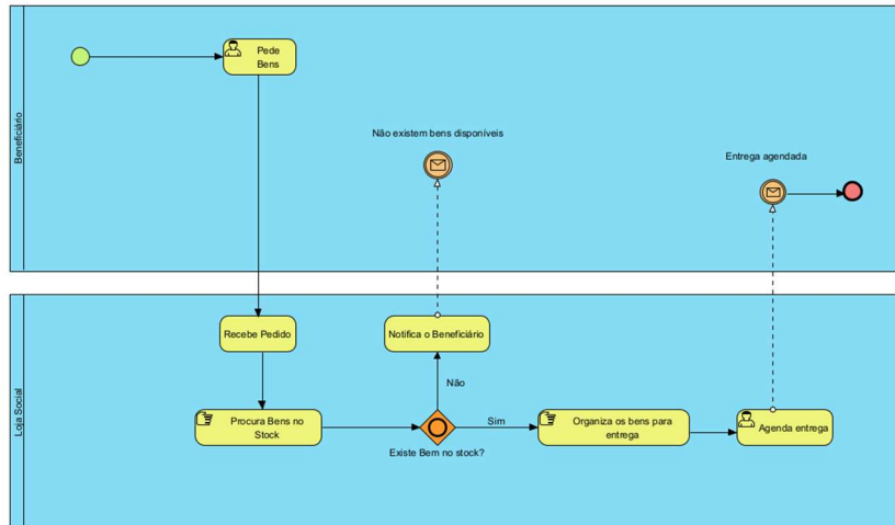
Figura 2 - Diagrama BPMN Pedir Apoio
