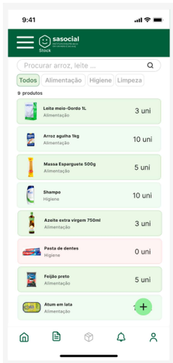
Figura 33– Mockup da página de stock
