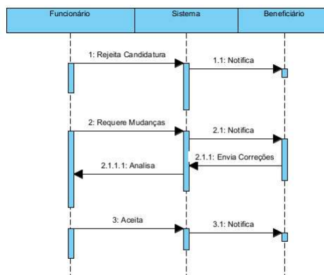
Figura 28 - Diagrama Sequência de Estado da Candidatura
