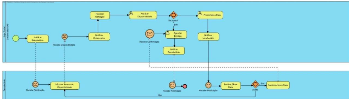
Figura 4 - Diagrama BPMN Agendamento De Entregas
