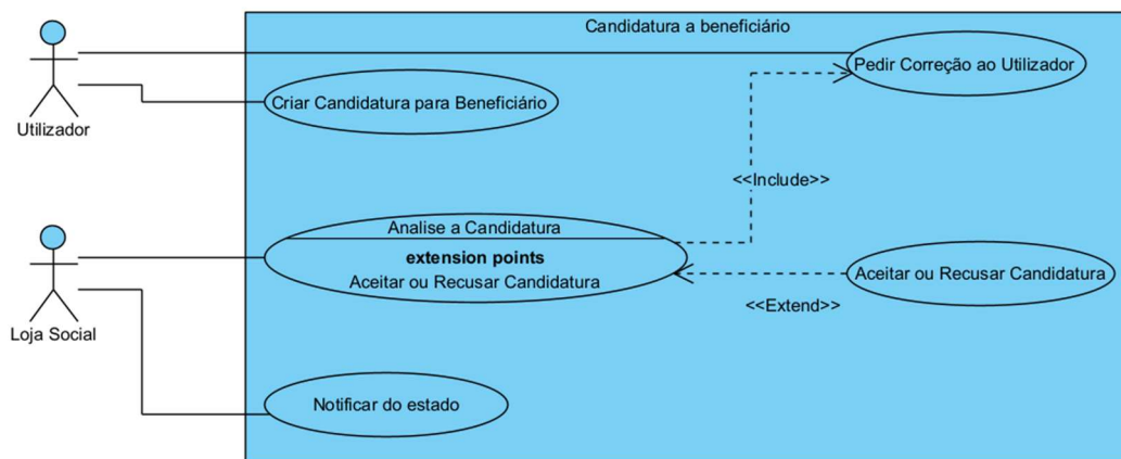
Figura 11 - Diagrama de Casos de Uso de Candidatura
