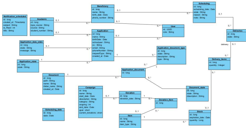
Figura 16- Diagrama de Classes
