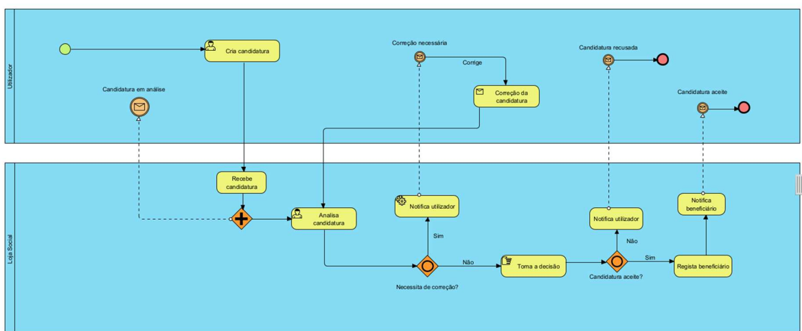
Figura 1 - Diagrama BPMN Candidatura
