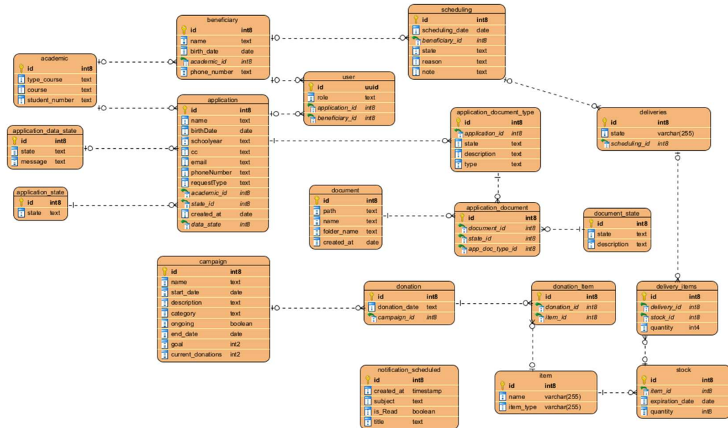
Figura 15 - Diagrama Entidade-Relação
