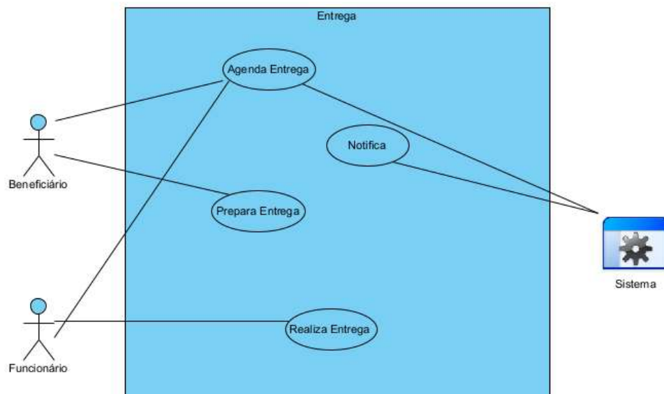
Figura 13 - Diagrama de Casos de Uso da entrega de bens
