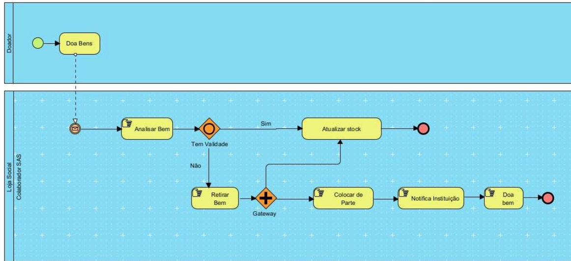
Figura 3 - Diagrama BPMN Gestão Inventário
