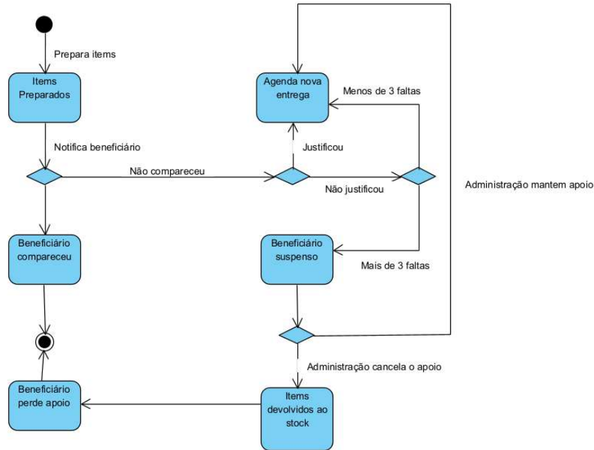
Figura 10 - Diagrama de Estados Gestão dos Beneficiários
