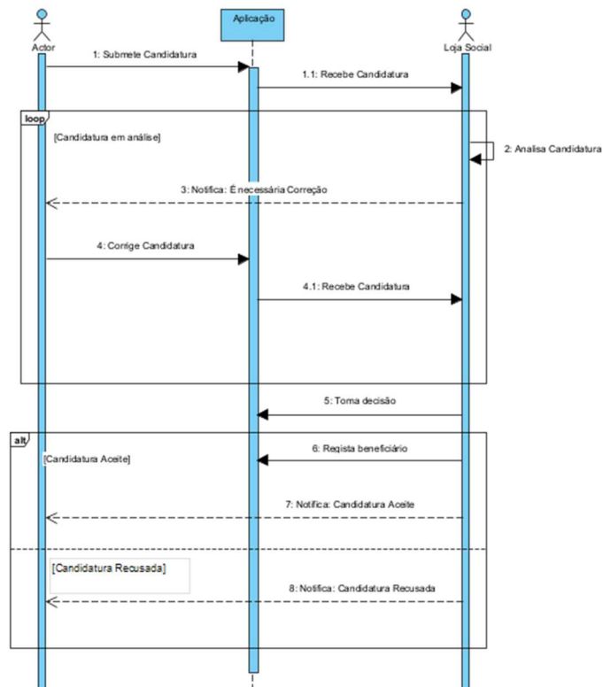
Figura 24 - Diagrama Sequência da Criação de Candidatura
