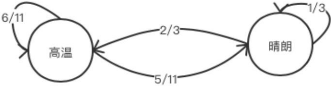
图 10 关卡三的天气跳转问题的状态转移图
