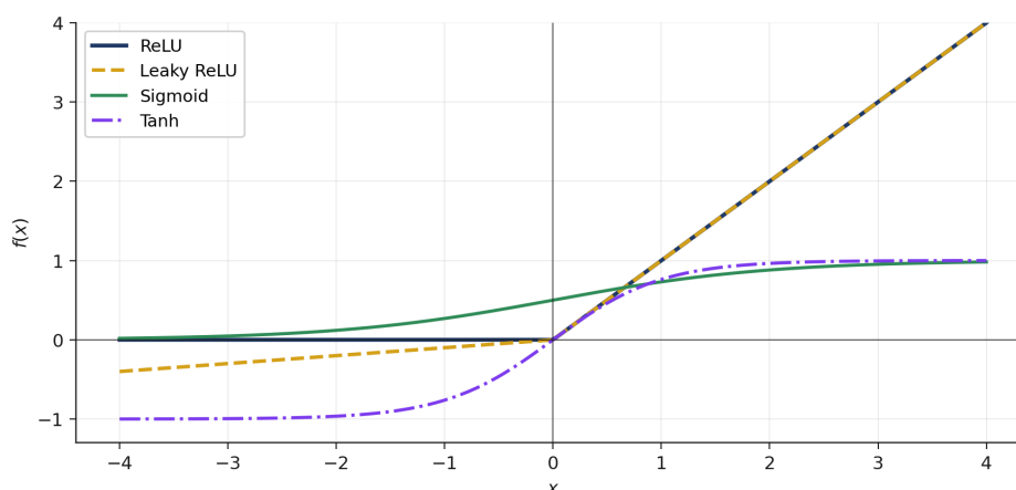
Figura 4. Funciones de activación habituales. ReLU es la más usada en capas convolucionales. Fuente: elaboración propia.
