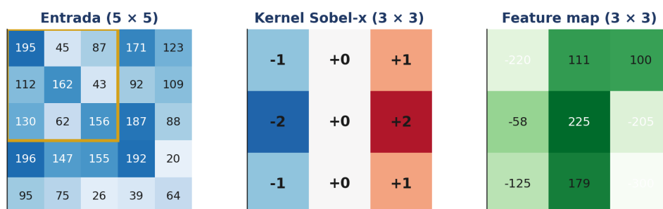
Figura 1. Operación de convolución: un filtro recorre la imagen y produce un mapa de características. Fuente: Stanford CS231n.
