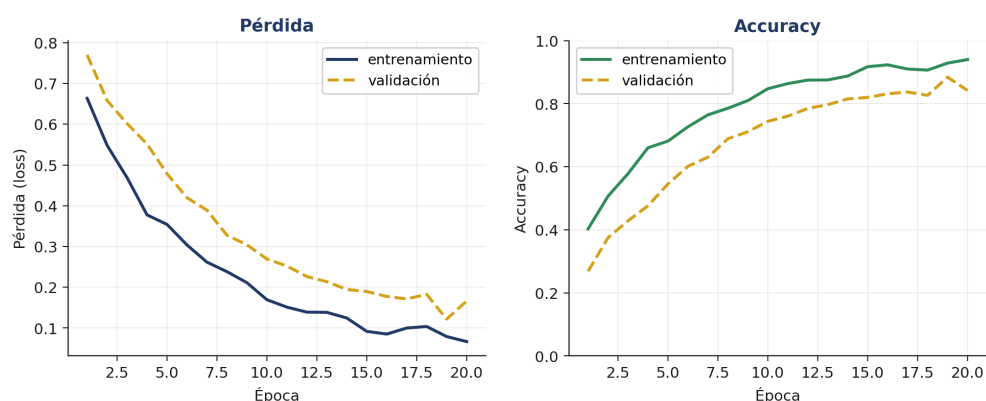
Figura 2. Curvas de aprendizaje esperadas sobre el dataset de botellas. Fuente: elaboración propia.
