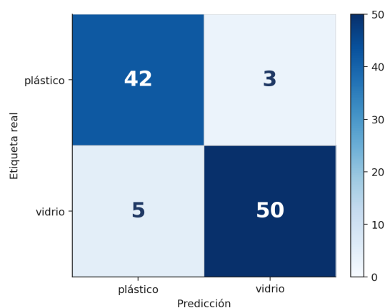
Figura 3. Matriz de confusión sobre validación: la diagonal son aciertos. Fuente: elaboración propia.
