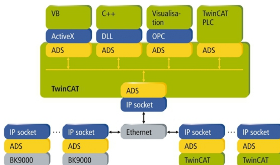
Figura 5. Arquitectura del protocolo ADS: las aplicaciones cliente acceden a las variables del PLC a través del router de TwinCAT. Fuente: Beckhoff Automation.
