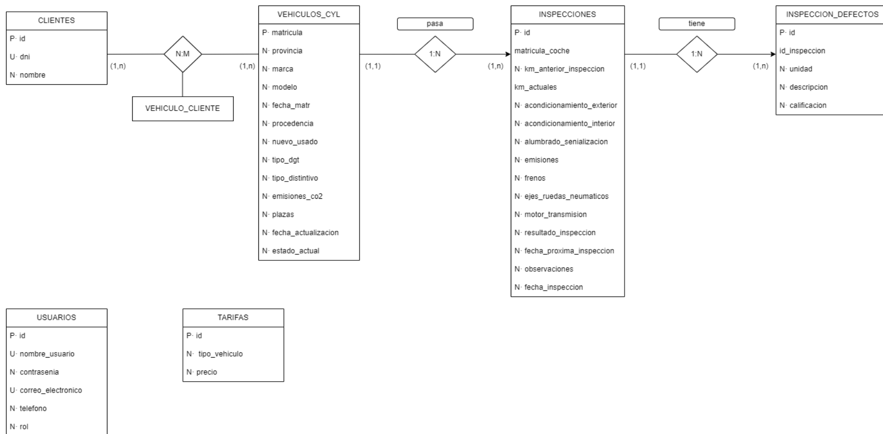
Ilustración 2. Diagrama Entidad-Relación
