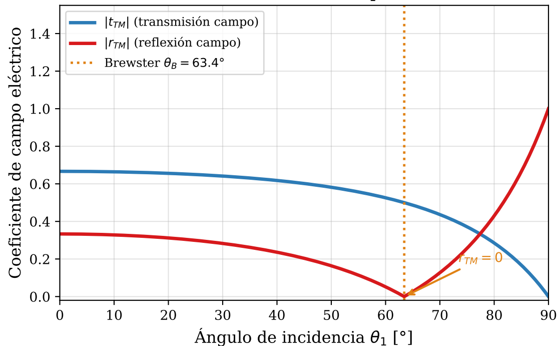
(b) Coeficientes de Campo — TM
