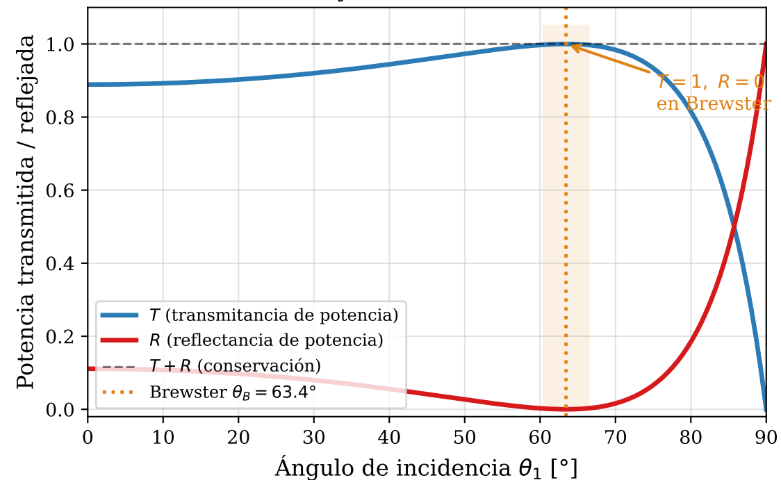
(a) Transmitancia y Reflectancia de Potencia — TM
