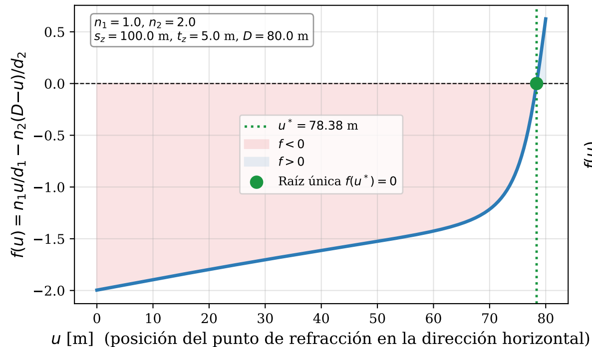
(a) Función de Snell 1D — monótona creciente
