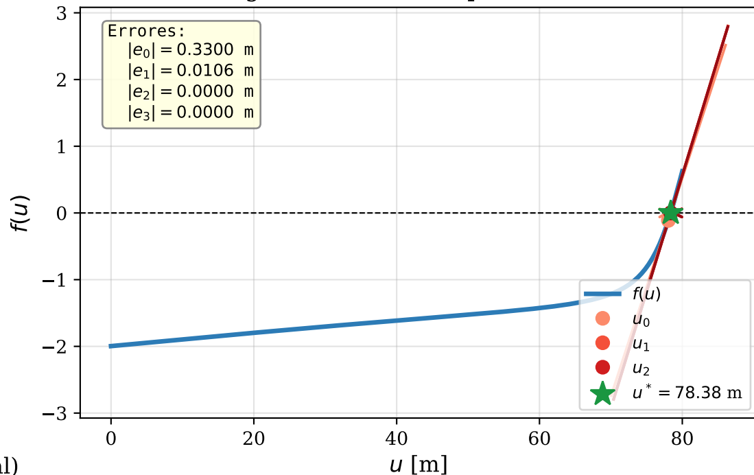
(b) Convergencia Newton-Raphson (4 iteraciones)
