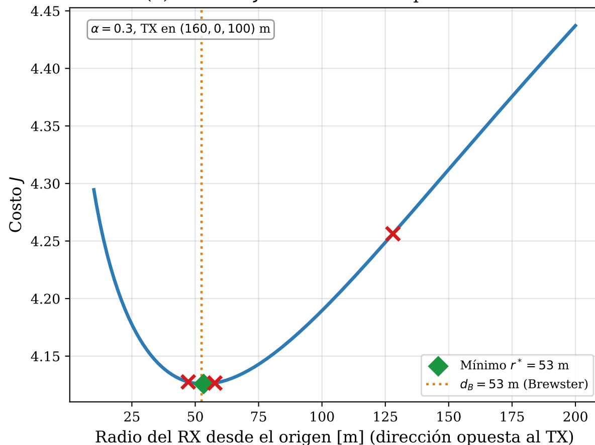
(b) Perfil de J en la dirección opuesta al TX
