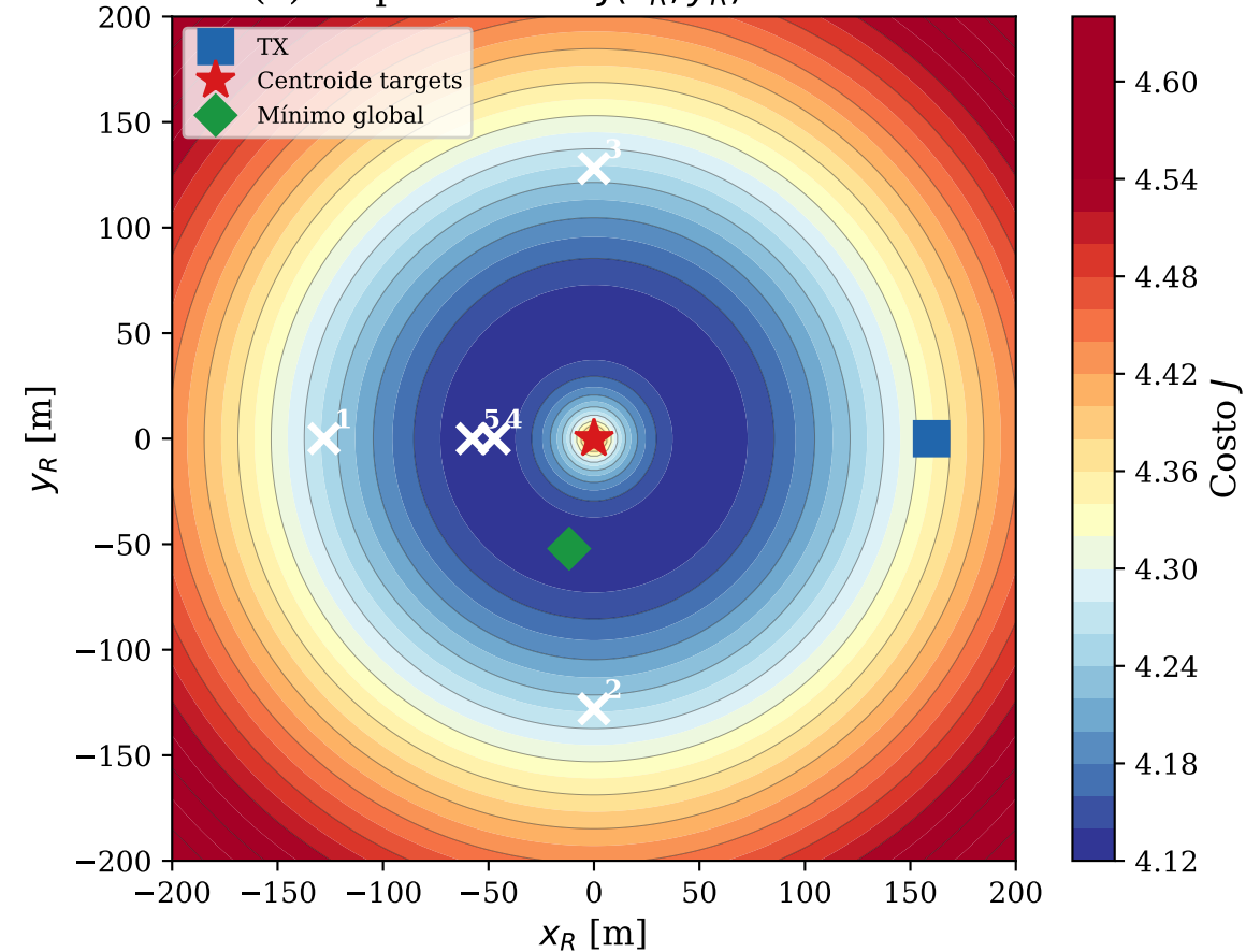
(a) Mapa de costo J(x_R, y_R) - \alpha = 0.3
