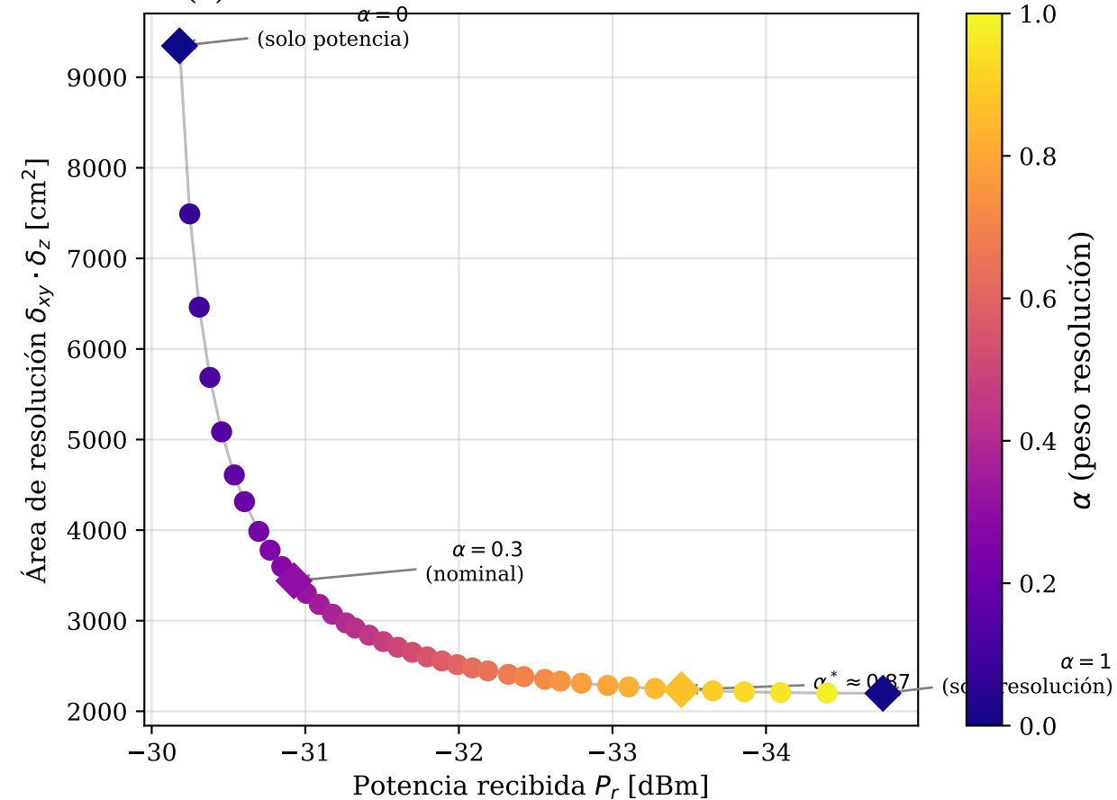
(a) Frontera de Pareto: Potencia vs. Resolución
