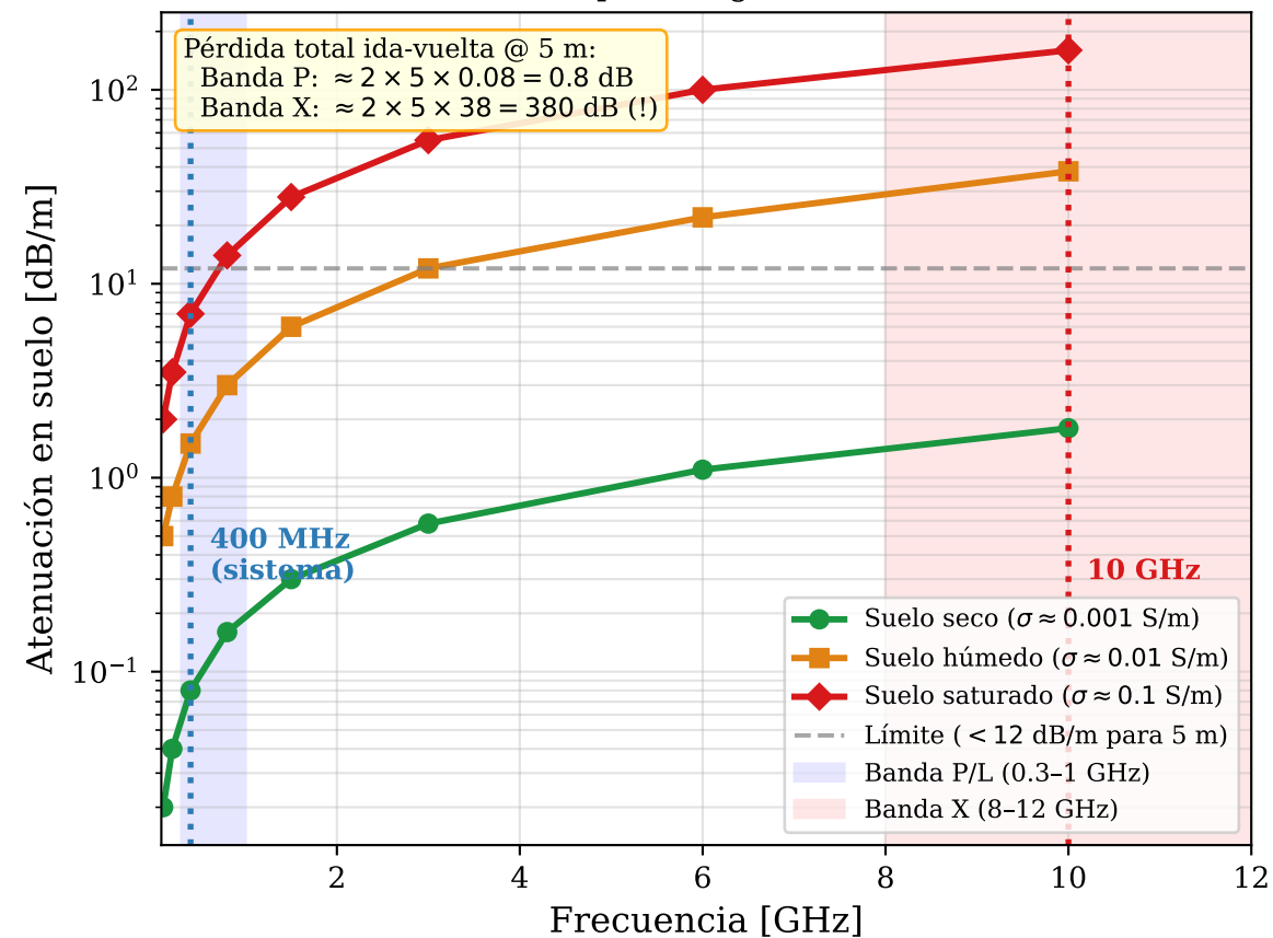
(a) Atenuación EM en suelo vs. frecuencia (razón para elegir banda P)
