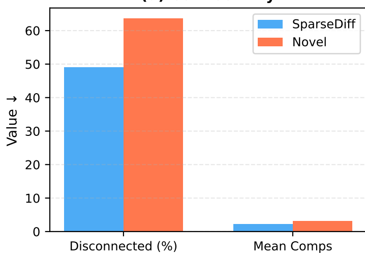
(d) Connectivity
