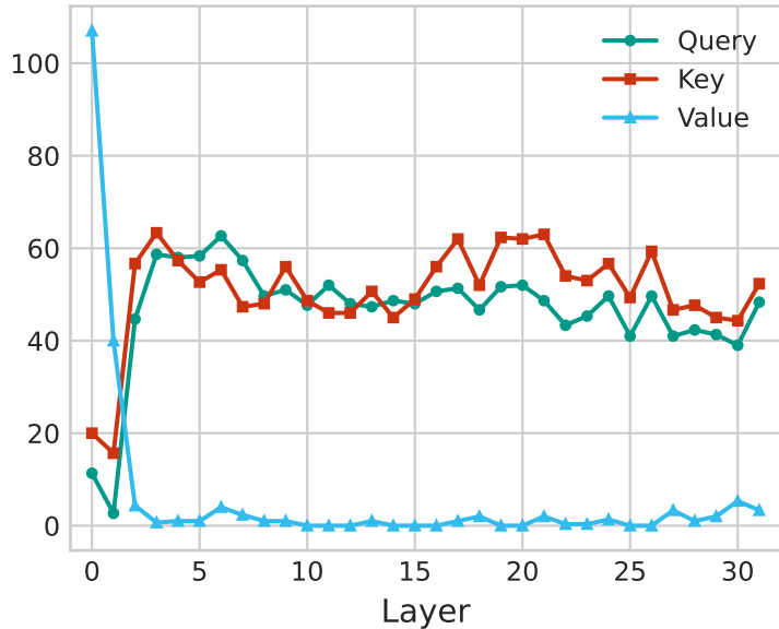
Llama-2-7B with RoPE
