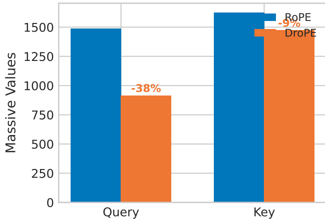
A. Massive Value Count (Llama-2-7B)
