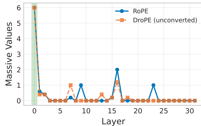
Value (V)
