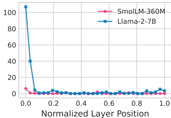
Value (V)
