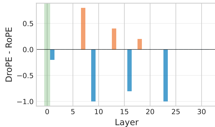
Value \Delta
