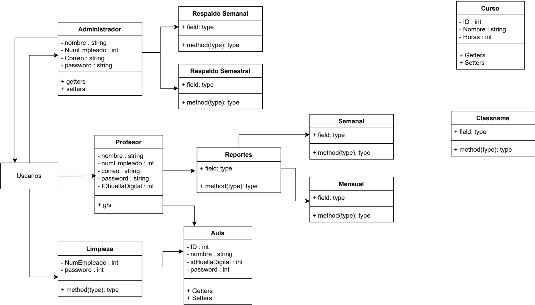
Diagrama de Clases
