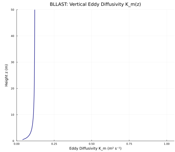
(d) BLLAST K_m(z) Credibility Ribbon
