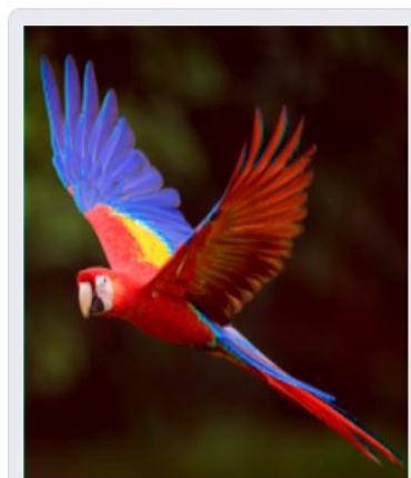
Activation Maximisation
