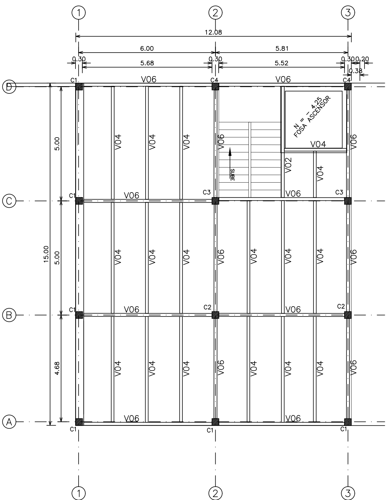
LOSA Nivel +0.00 Escala 1:100
