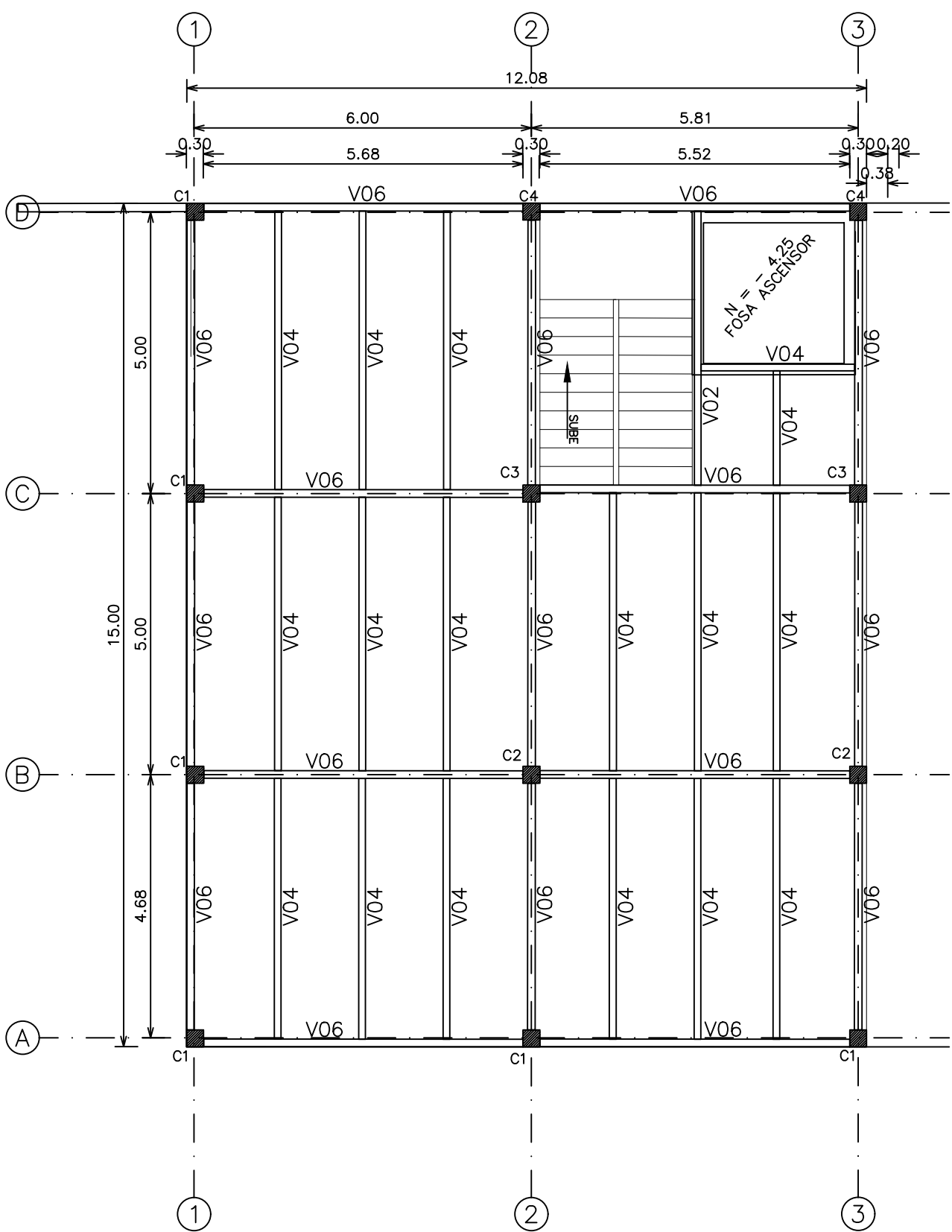
LOSA Nivel +3.40; +6.20 Escala 1:100
