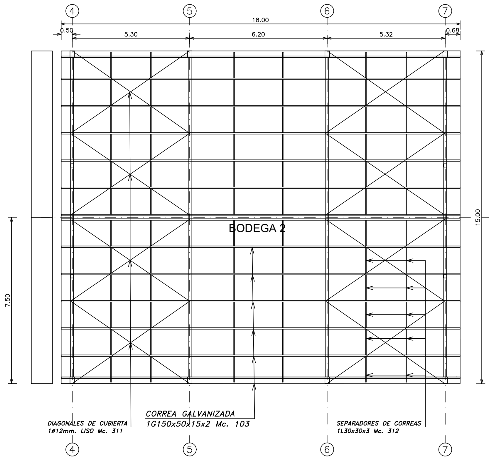
CUBIERTA BODEGA 2 Escala 1:100
