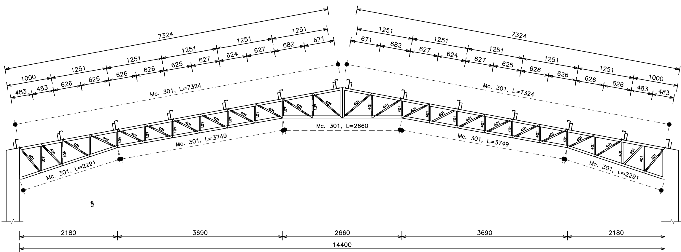
DETALLE DE VIGA TIPO 1 Escala 1:50
