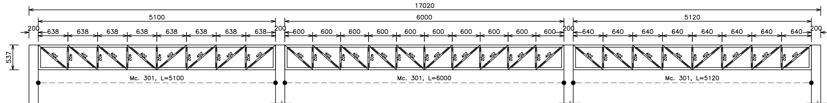
DETALLE DE VIGA TIPO 2 Escala 1:50
