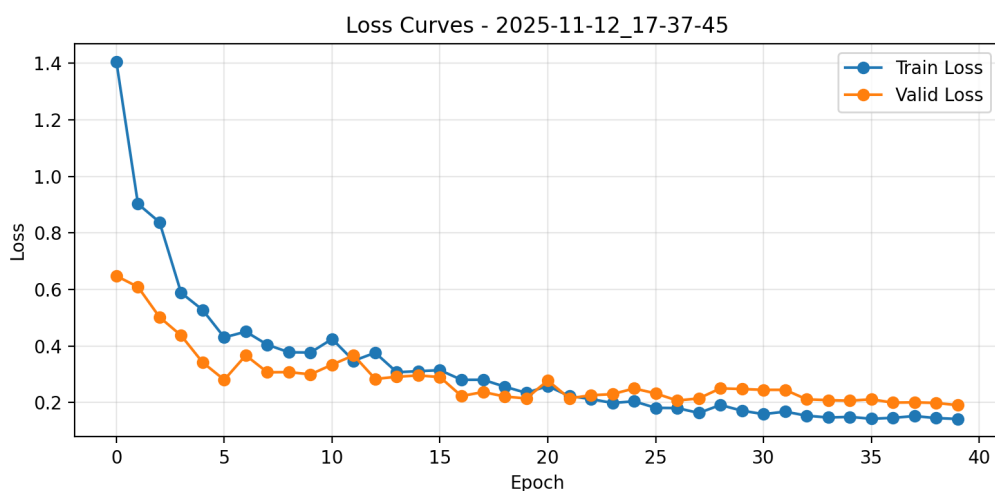
图 1: 鸟巢检测训练/验证损失曲线；约第 20 轮后趋于平稳。
