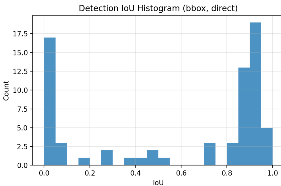
图 3: 鸟巢检测 bbox IoU 分布; 右偏表明定位质量较好。
