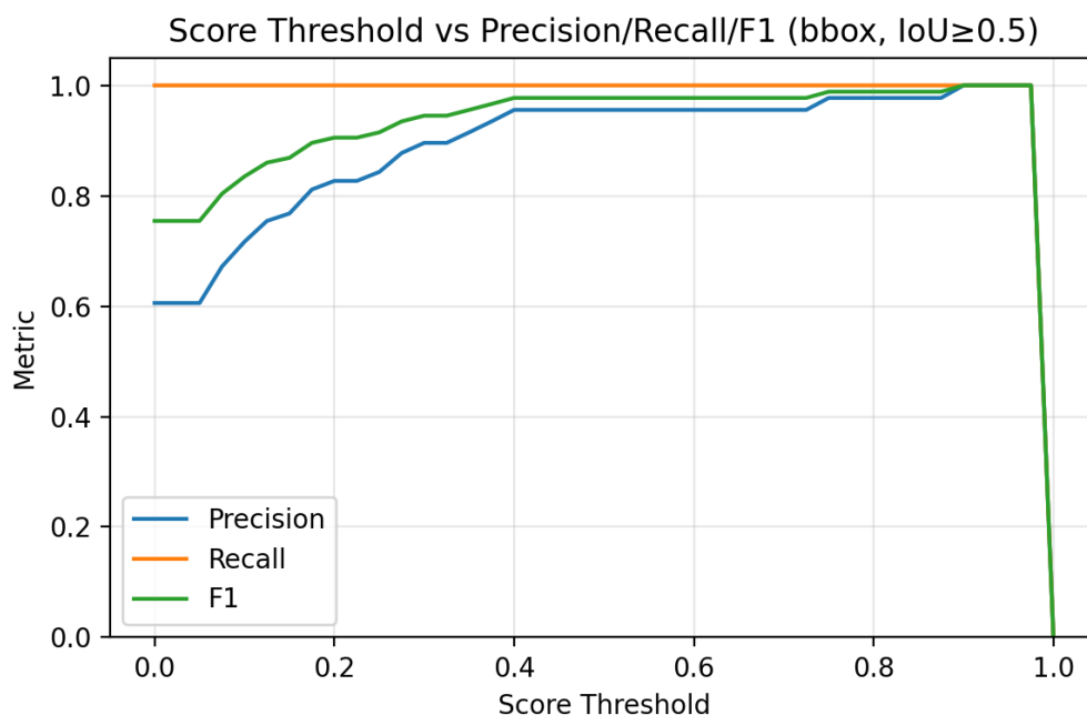
图 4: 得分阈值与精确率/召回率/F1 关系 ( \text{IoU} \geq 0.5 ); 阈值 0.4–0.5 附近 F1 较优。
