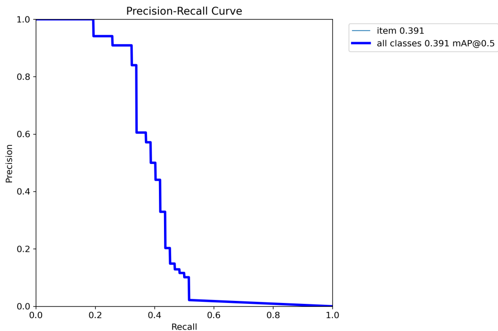
图 5: 漏油检测 (train10-csdcn) 验证集精确率-召回率曲线; IoU 阈值 0.5。
