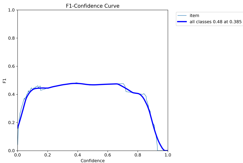
图 6: 漏油检测 (train10-csdcn) 验证集 F1 曲线; 不同置信度阈值下的 F1 分数。
