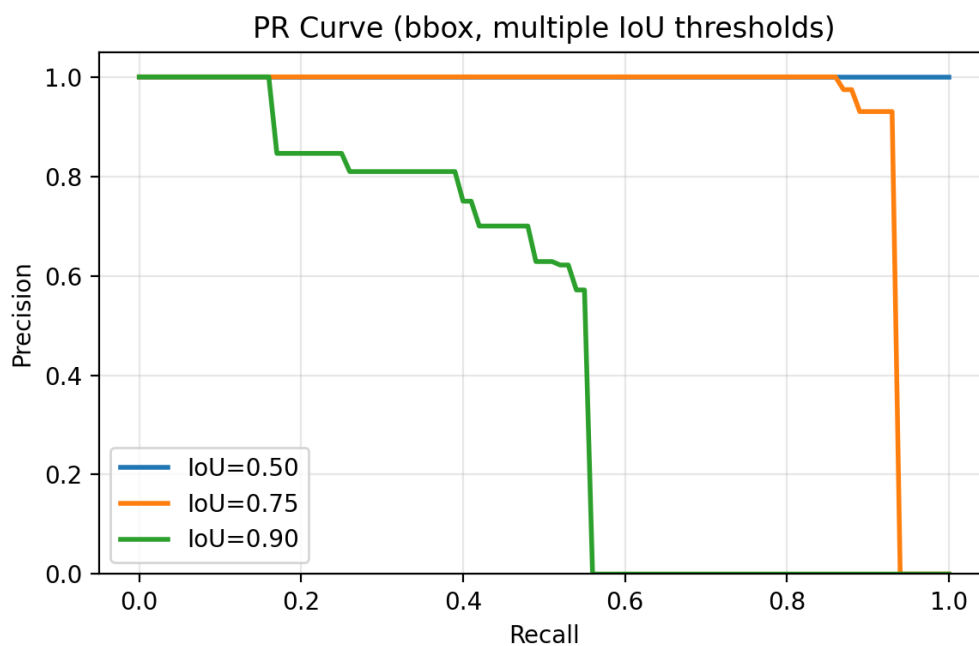
图 2: 鸟巢检测 bbox PR 曲线 (IoU 0.50/0.75/0.90)。
