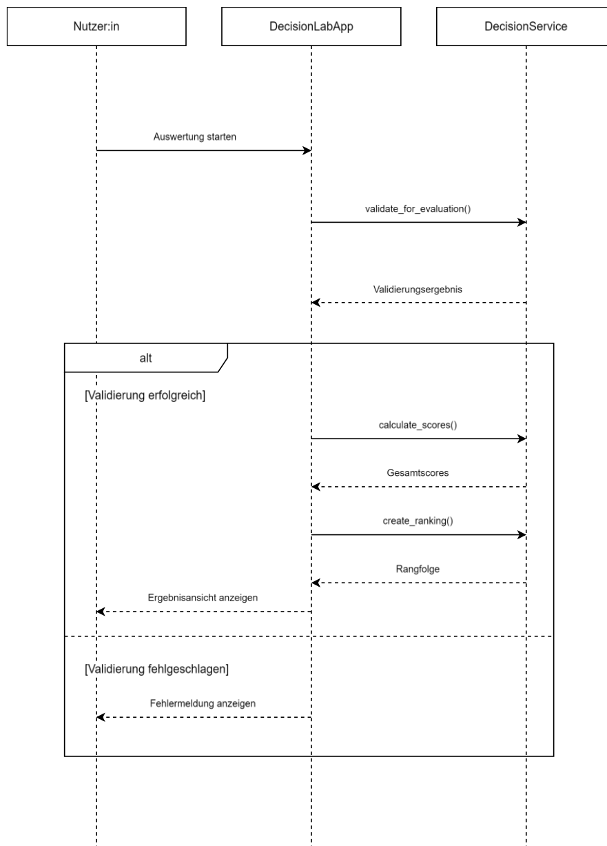
Abbildung 3: UML-Sequenzdiagramm "Auswertung durchführen"
