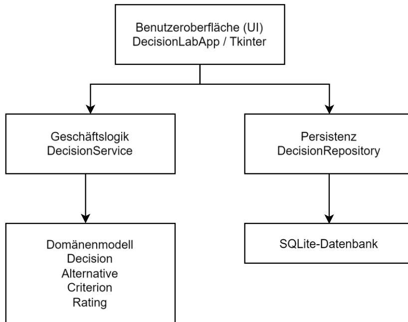
Abbildung 1: Architekturübersicht von DecisionLab
