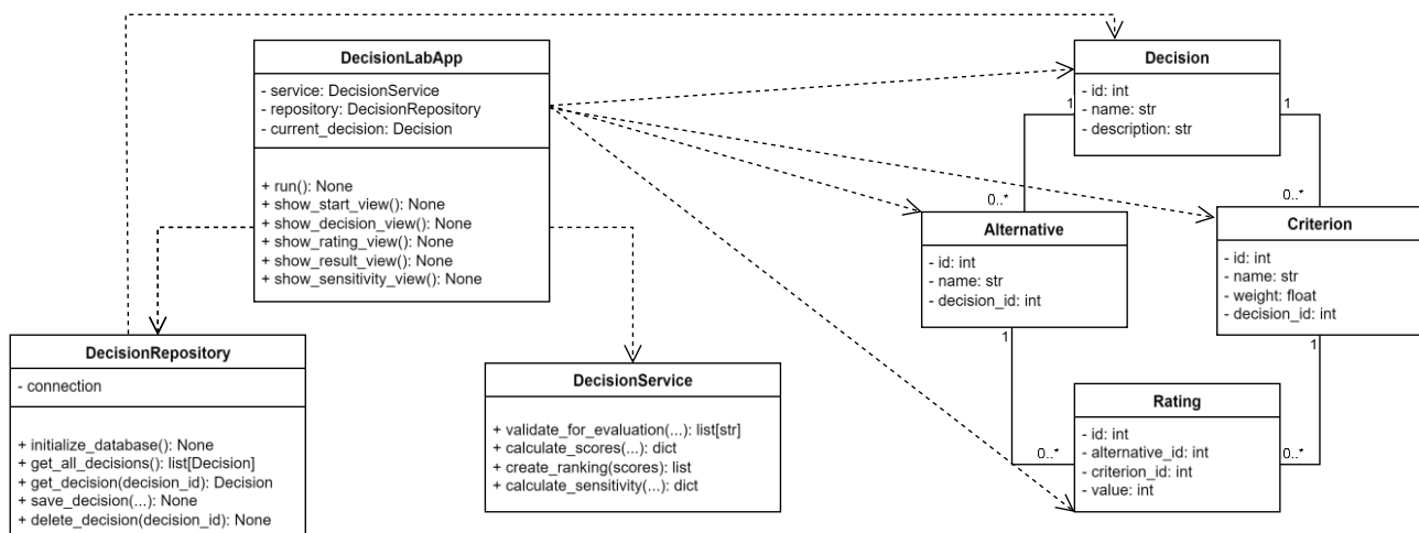
Abbildung 2: UML-Klassendiagramm der Softwarearchitektur von DecisionLab
